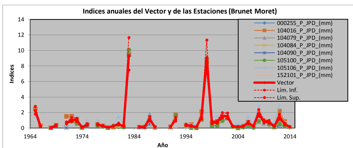
Figura 7. Vector regional de la precipitación con las mejores estaciones del Grupo 2
