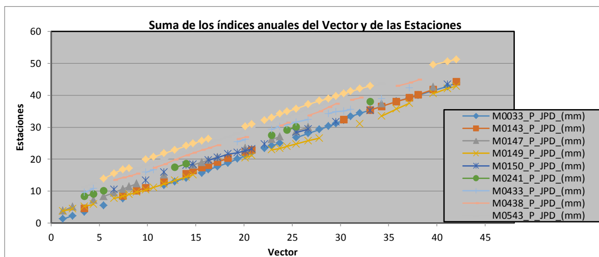
Figura 14. Curva de doble masa de índices de precipitación de las mejores estaciones del Grupo 5
