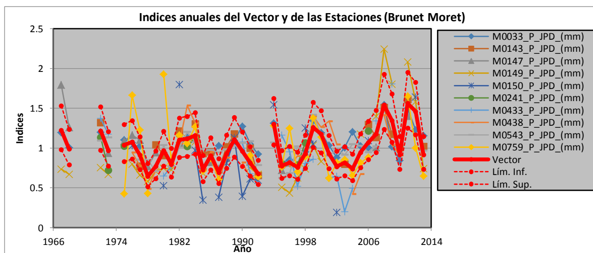
Figura 13. Vector regional de la precipitación de las mejores estaciones del Grupo 5
