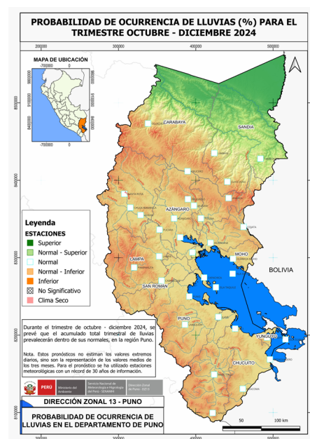
Figura 10: Pronóstico de lluvias entre octubre a diciembre de 2024
