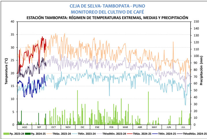
Figura 4: Temperaturas máxima, mínima, para el Cultivo Café - campaña 2024-2025 en la Estación CO. Tambopata
