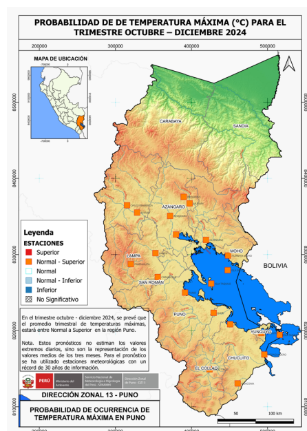
Figura 8: Pronóstico de temperatura máxima entre octubre a diciembre de 2024
