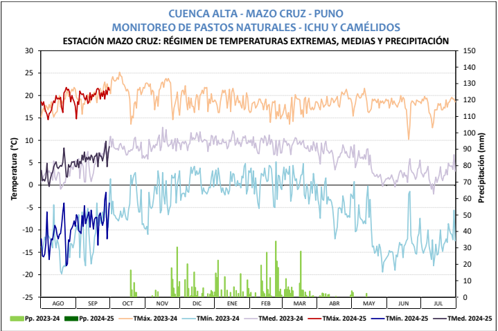
Figura 6: Temperaturas máxima, mínima, umbrales óptimos y críticos para pastos naturales - el ichu-campaña 2024-2025 en la Estación CO. Mazocruz
