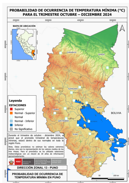
Figura 9: Pronóstico de temperatura mínima entre octubre a diciembre de 2024
