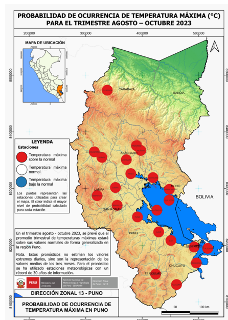
Figura 8: Pronóstico de temperatura máxima de agosto a octubre de 2023
