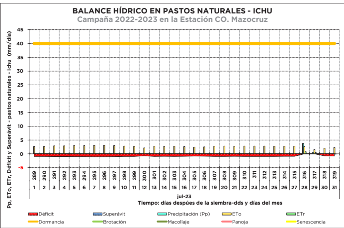
Figura 7: Balance hídrico diario para pastos naturales - el ichu - campaña 2022-2023 en la Estación CO. Mazocruz
