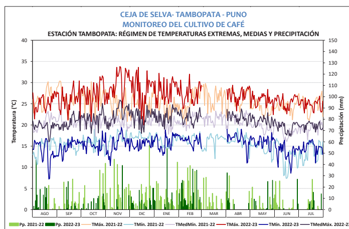
Figura 4: Temperaturas máxima, mínima, para el Cultivo Café - campaña 2022-2023 en la Estación CO. Tambopata
