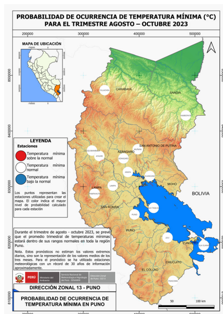
Figura 9: Pronóstico de temperatura mínima de agosto a octubre de 2023
