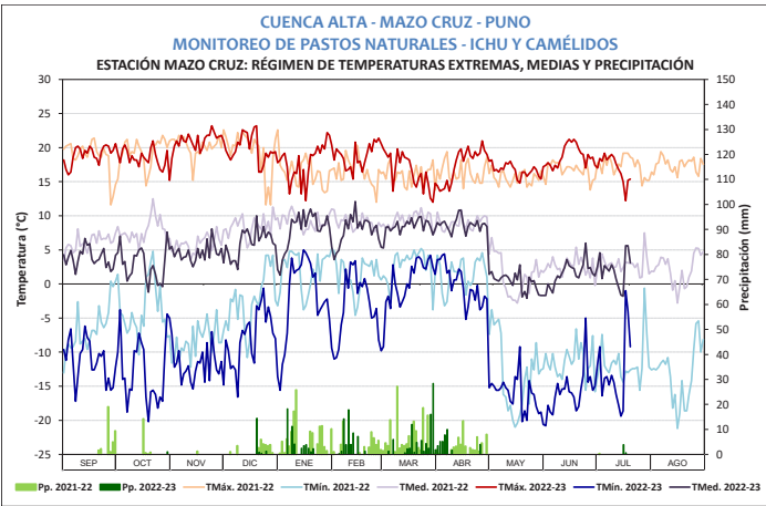
Figura 6: Temperaturas máxima, mínima, umbrales óptimos y críticos para pastos naturales - el ichu-campaña 2022-2023 en la Estación CO. Mazocruz
