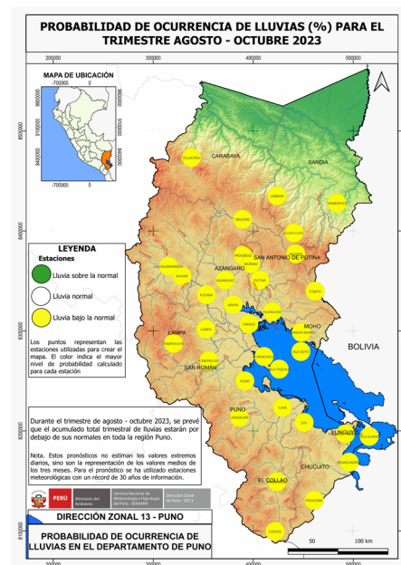
Figura 10: Pronóstico de lluvias de agosto a octubre de 2023
