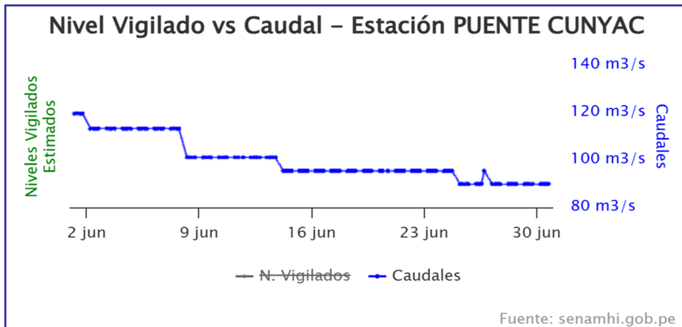
Figura 14. Hidrograma estación Cunyac mes de junio del 2025
