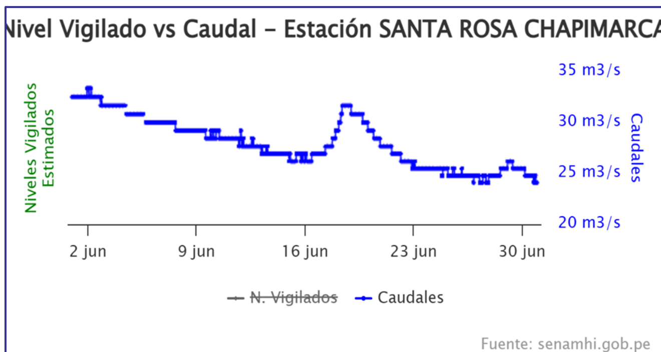
Figura 15. Hidrograma estación Santa Rosa mes de junio del 2025
