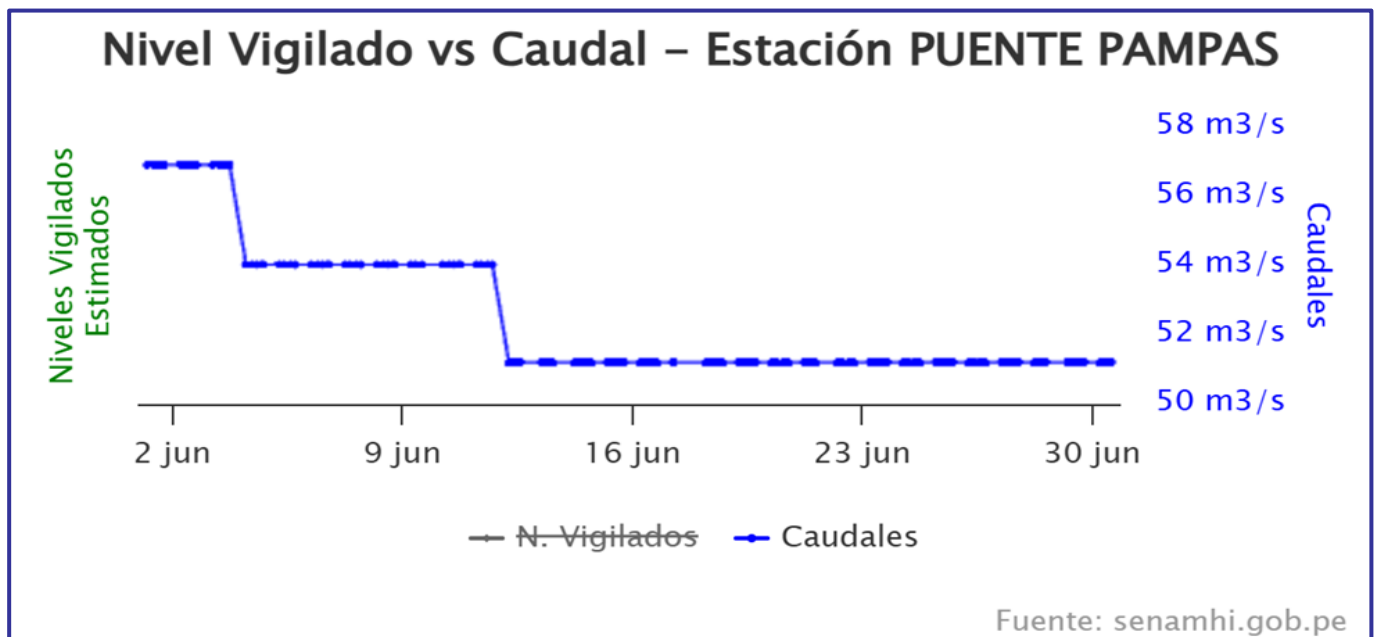
Figura 17. Hidrograma estación Puente Pampas mes de junio del 2025
