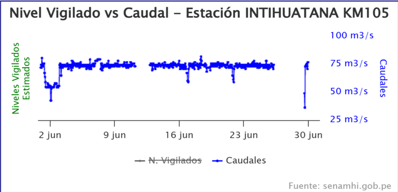
Figura 10. Hidrograma estación Intihuatana km 105 mes de junio del 2025
