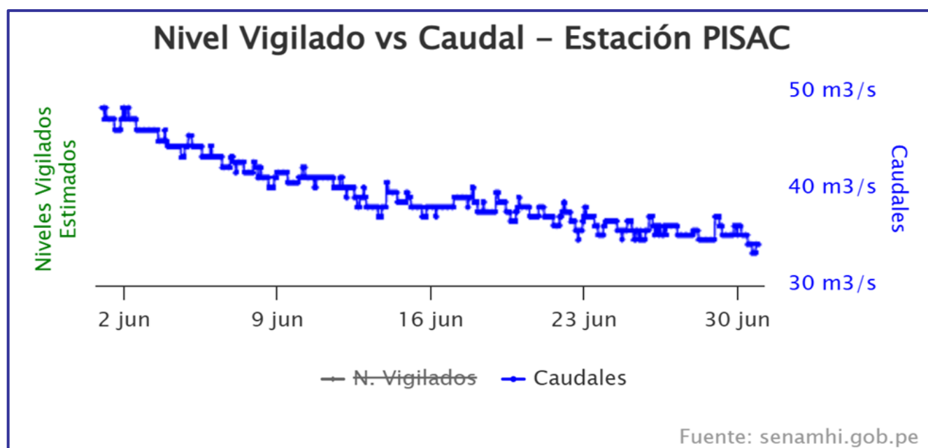
Figura 8. Hidrograma estación Pisac mes de junio del 2025
