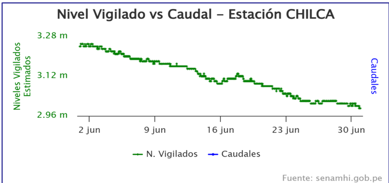
Figura 9. Hidrograma estación Chilca mes de junio del 2025
