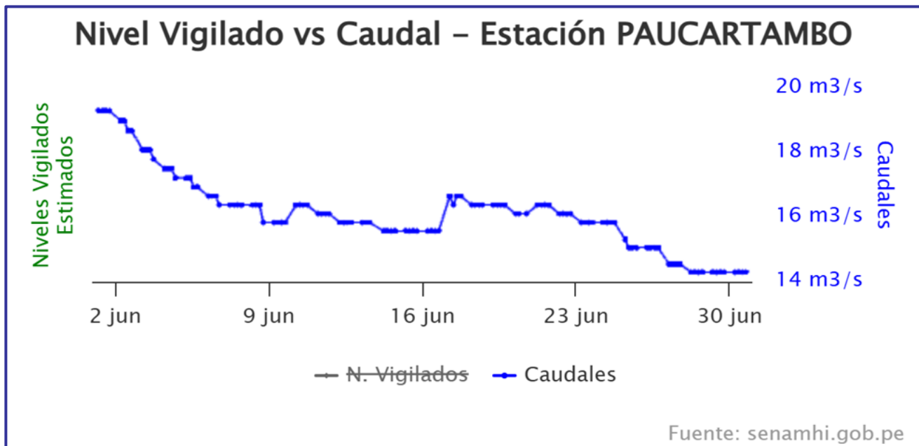
Figura 12. Hidrograma estación Paucartambo mes de junio del 2025
