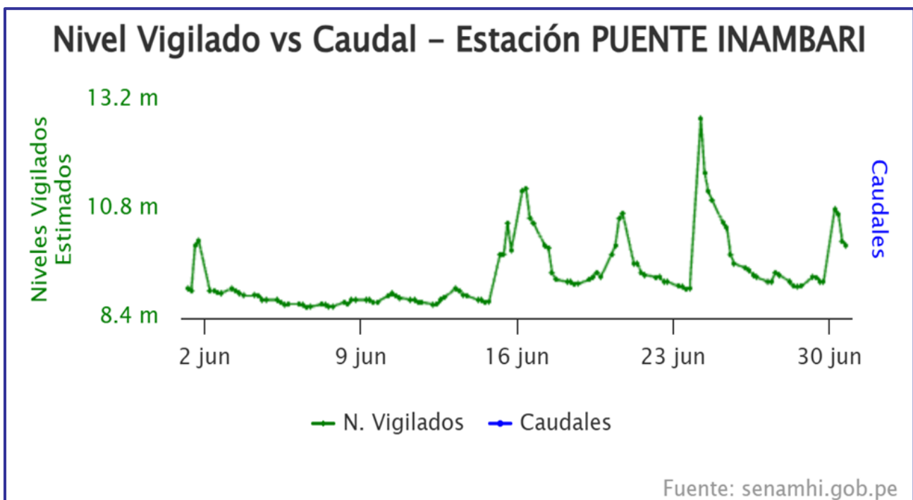
Figura 19. Hidrograma estación Río Inambari mes de junio del 2025
