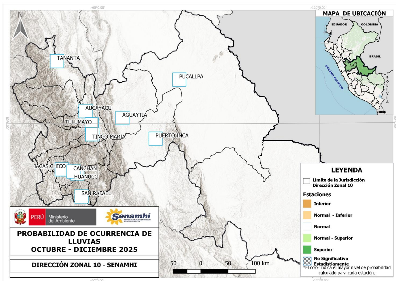
Figura3. Pronóstico de lluvias para el trimestre octubre - diciembre 2025. Fuente: DZ10-SENAMHI
