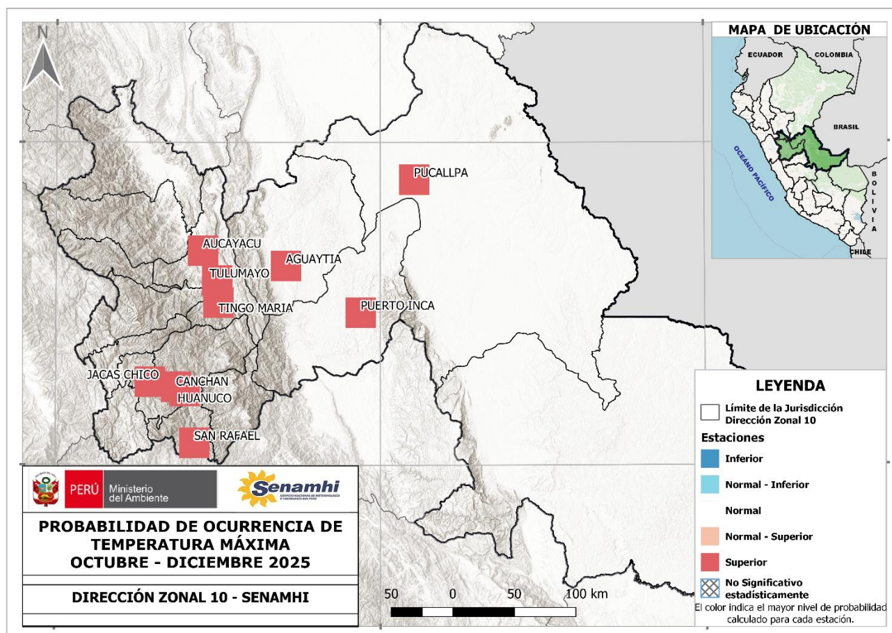
Figura1. Probabilidad de ocurrencia de temperaturas máximas para el trimestre octubre - diciembre 2025.
