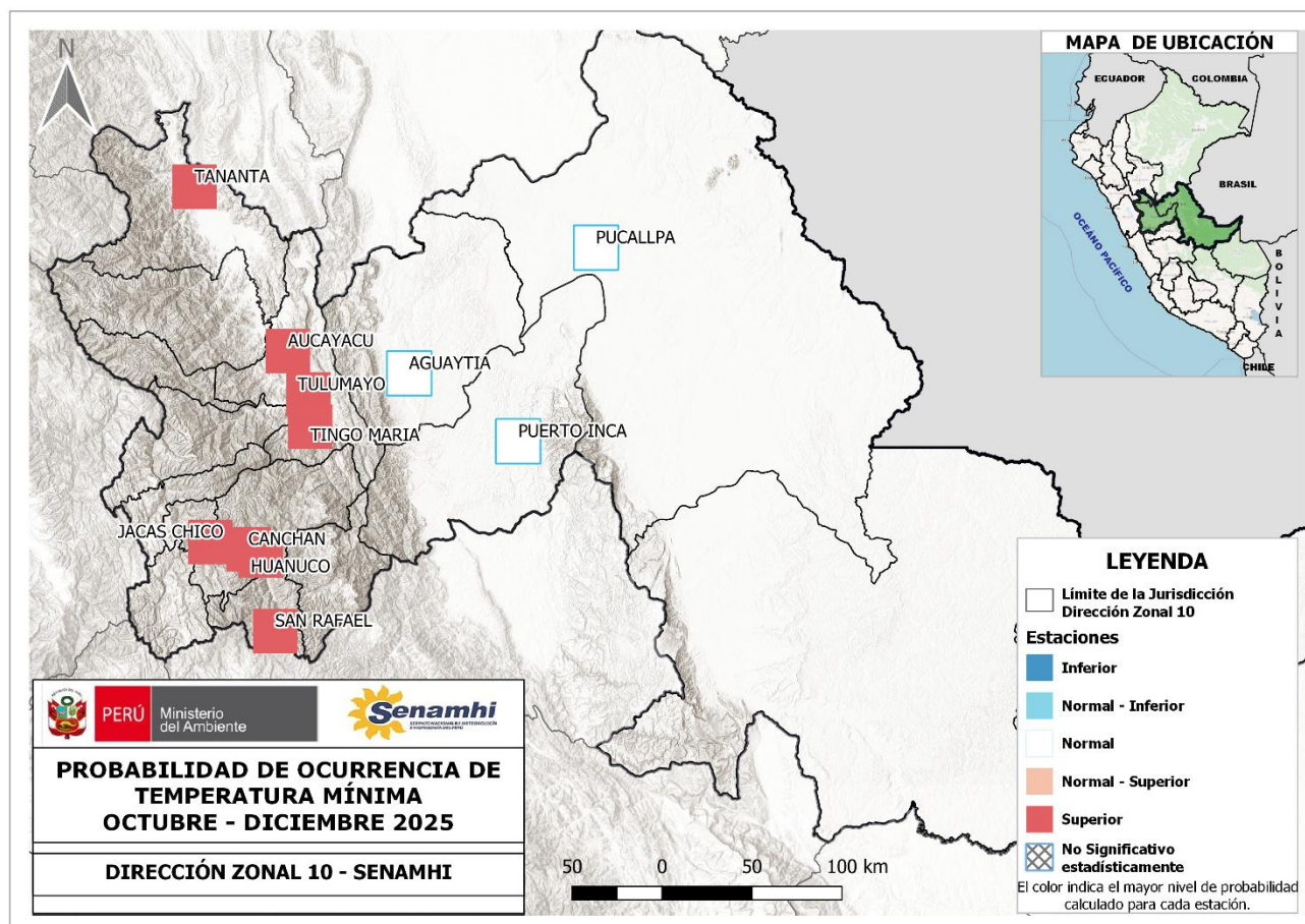
Figura2. Probabilidad de ocurrencia de temperaturas mínimas para el trimestre octubre - diciembre 2025.
