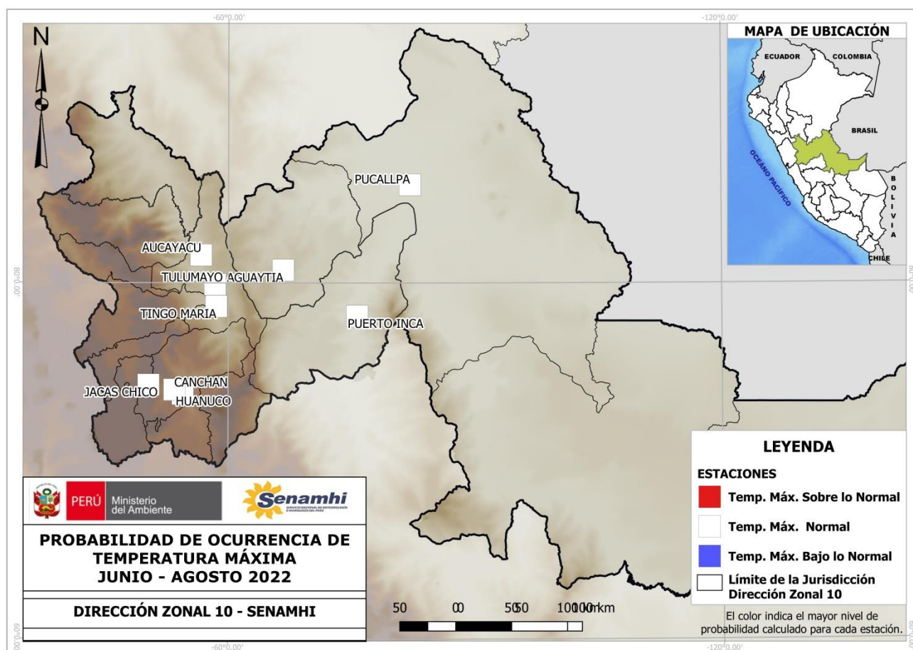
Figura1. Probabilidad de ocurrencia de temperaturas máximas para el trimestre junio - agosto 2022. Fuente: DZ10-SENAMHI
