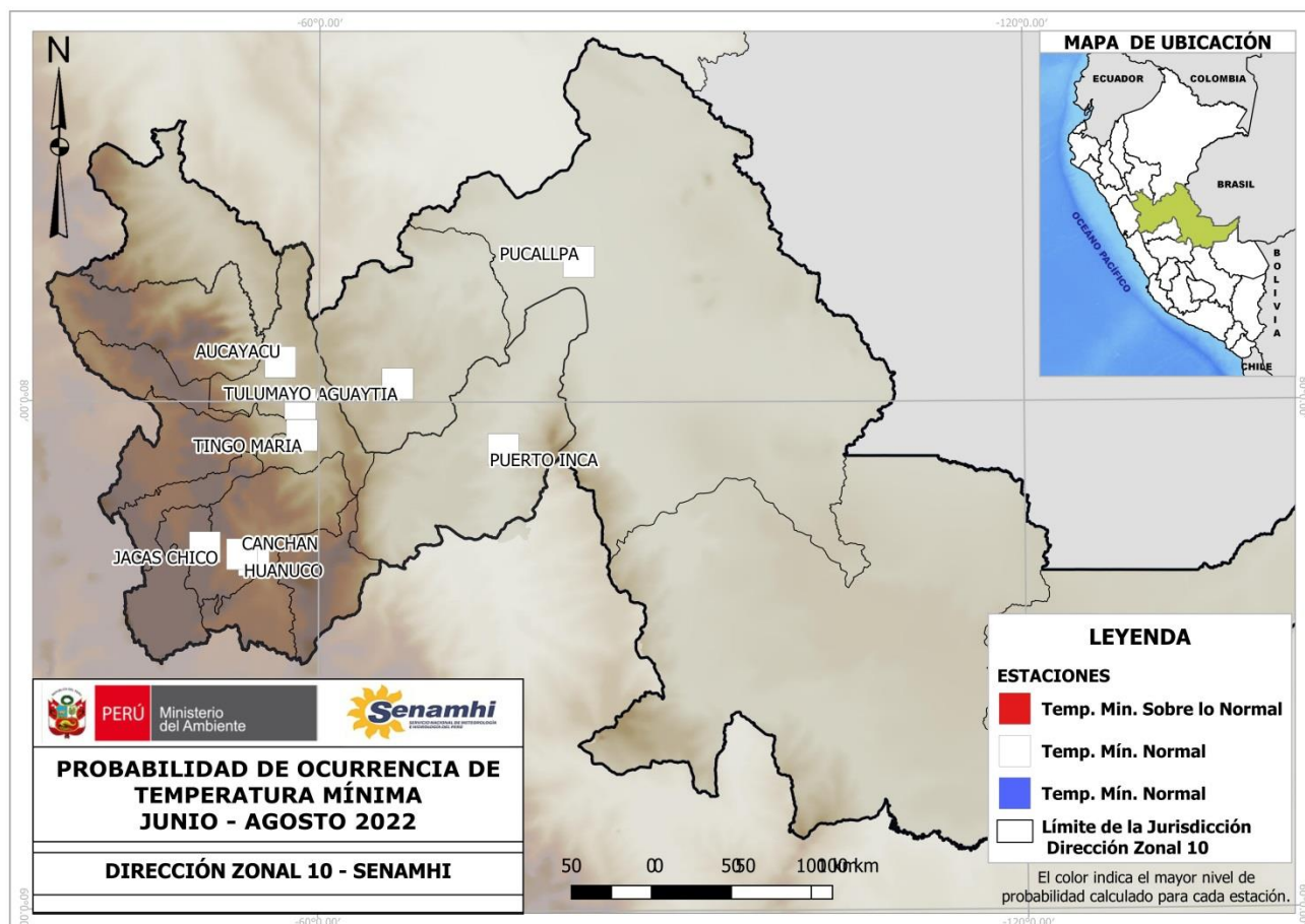
Figura2. Probabilidad de ocurrencia de temperaturas mínimas para el trimestre junio - agosto 2022. Fuente: DZ10-SENAMHI
