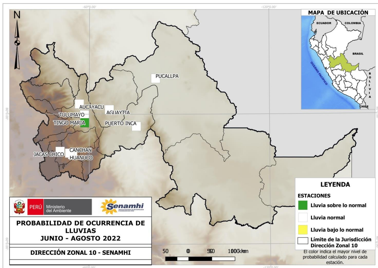
Figura3. Pronóstico de lluvias para el trimestre junio - agosto 2022. Fuente: DZ10-SENAMHI
