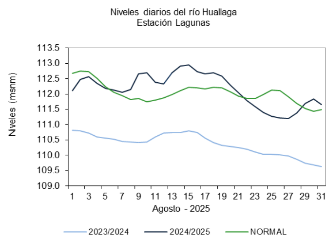
Gráfico 11. Hidrograma del río Huallaga. Estación HLM Lagunas
