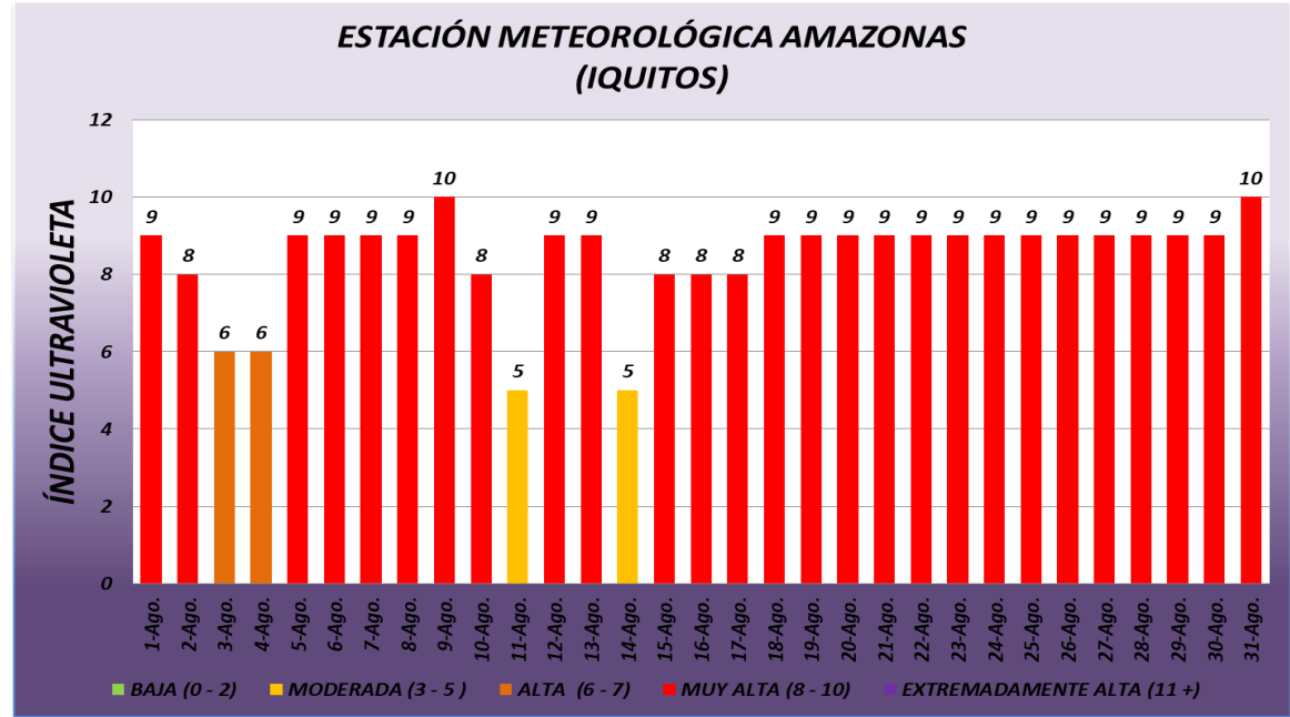
Gráfico 20. Índice Ultravioleta IUV de la Estación Amazonas, Iquitos, valor máximo durante el mes de Agosto del 2025.
