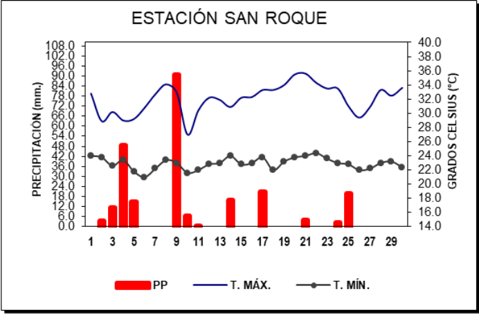
Gráfico 2. Termopluiometría de la estación CO-San Roque.
