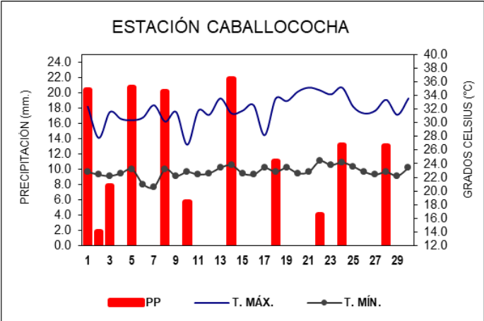
Gráfico 1. Termopluiometría de la estación CO-Cabalcocha.
