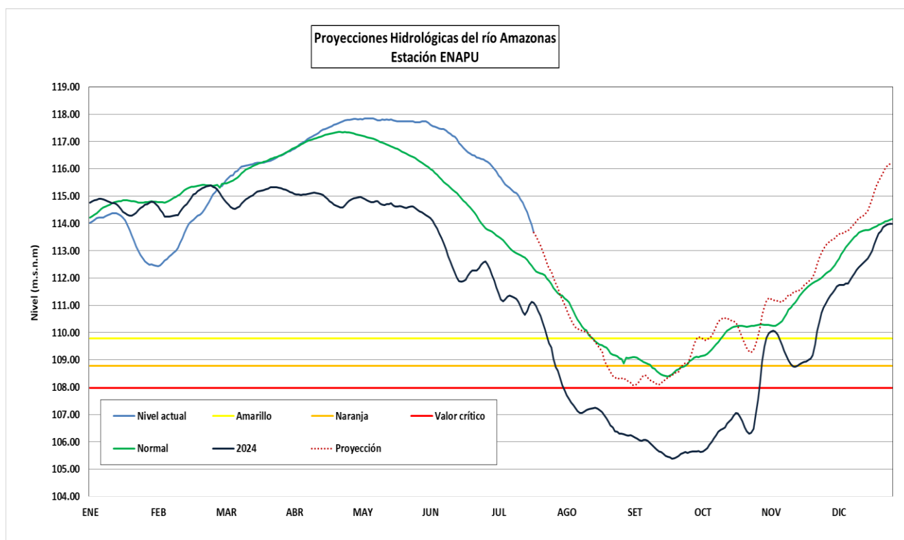
Gráfico 14. Comportamiento y tendencia del río Amazonas.
