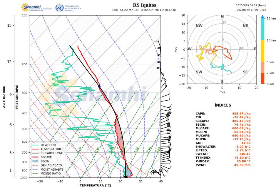
Gráfico 23. Perfil atmosférico de Iquitos, 29/08/2025.
