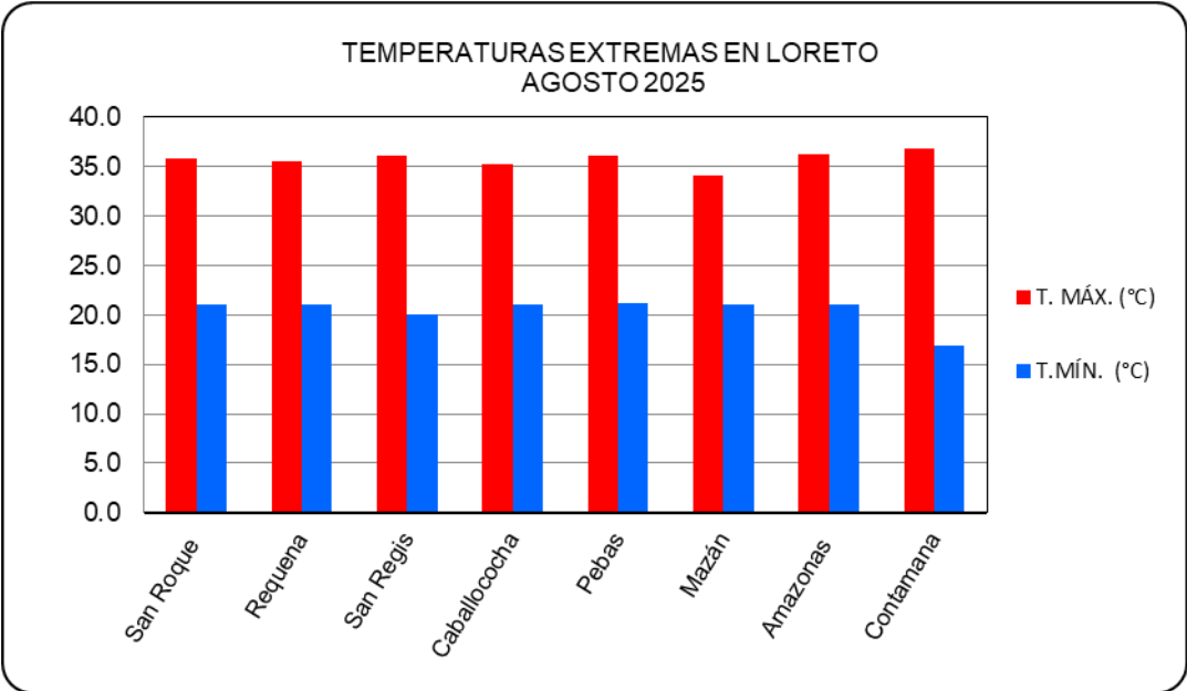
Gráfico 7. Temperaturas extremas en Loreto.
