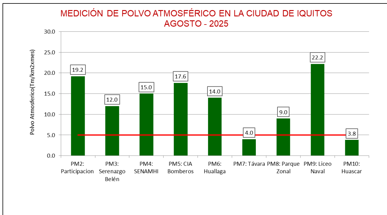
Gráfico 18. Resultados del monitoreo de los CSS en la ciudad de Iquitos durante el mes de Agosto 2025.
