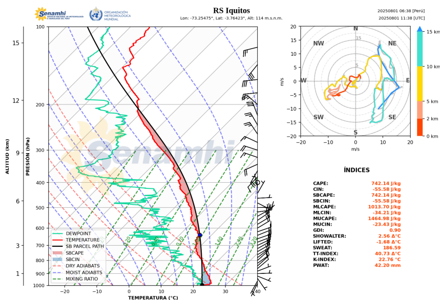
Gráfico 21. Perfil atmosférico de Iquitos, 01/08/2025.
