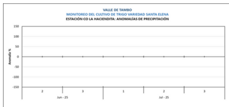
Gráfico Nro. 06. Muestra las anomalías de precipitación en la estación CO. La Haciendita.
