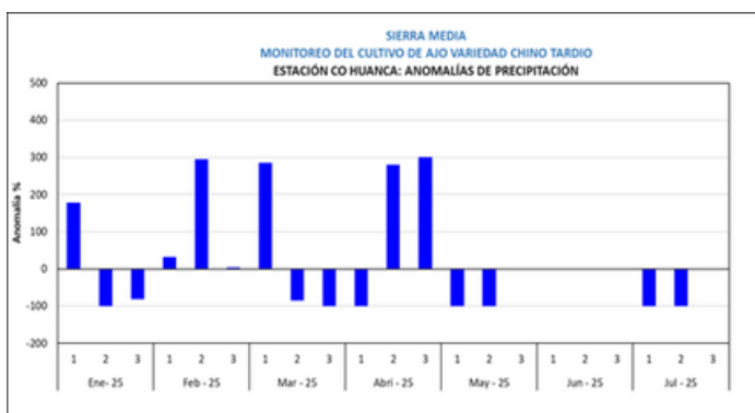
Gráfico Nro. 14. Muestra las anomalías de precipitación en la estación CO. Huanca.
