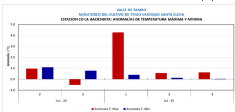
Gráfico Nro. 07. Muestra las anomalías de la temperatura máxima y mínima en la estación CO. La Haciendita.
