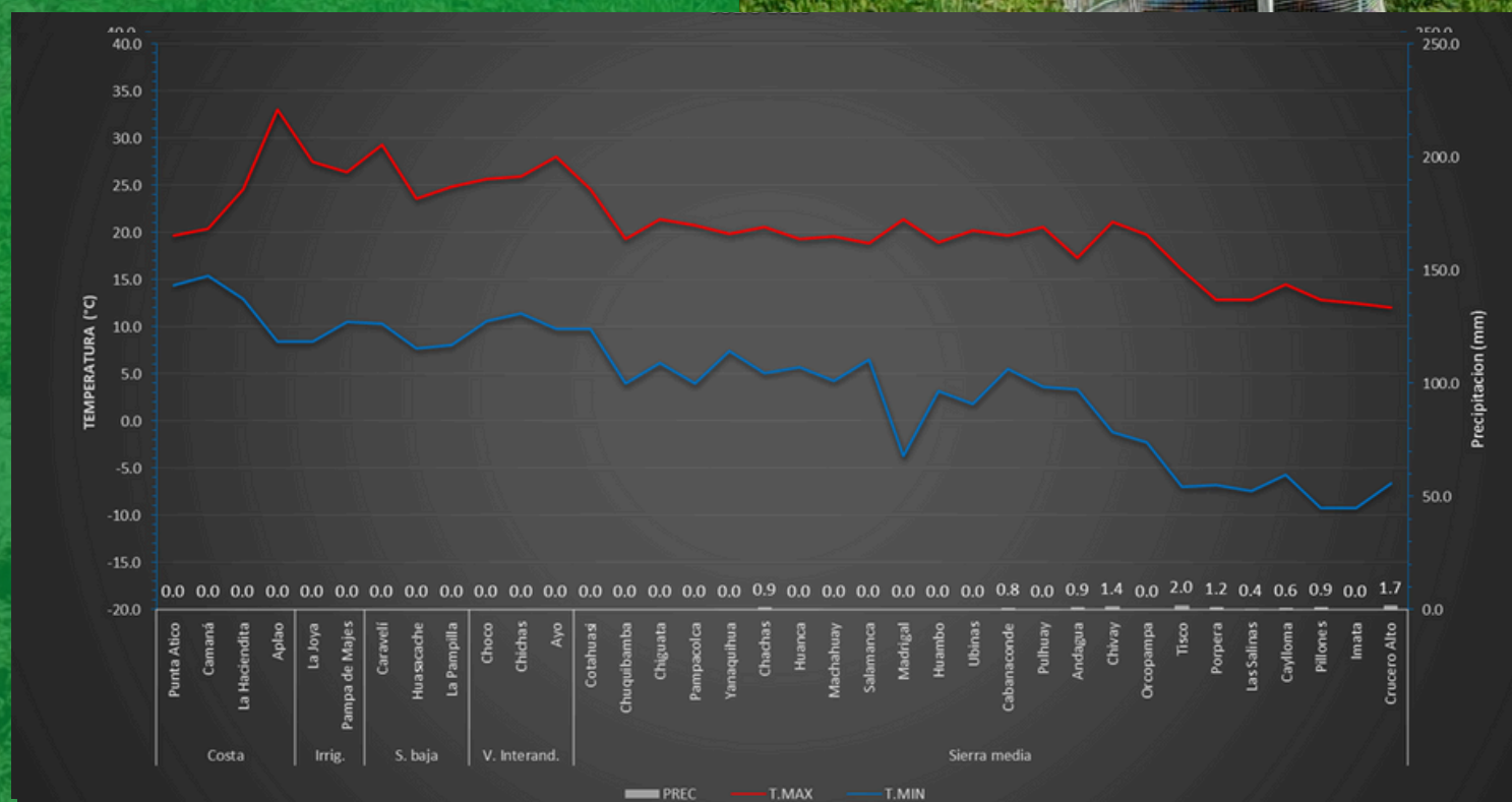
Temperaturas y precipitaciones por estaciones - julio 2025
