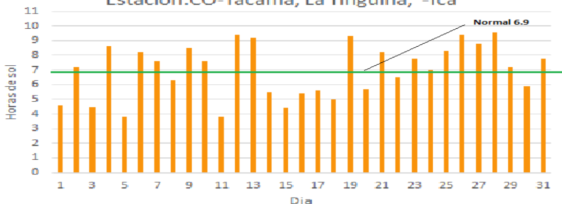
Fig.2: Horas de sol total diario julio 2021 Estacion: CO-Tacama, La Tinguña, -Ica
