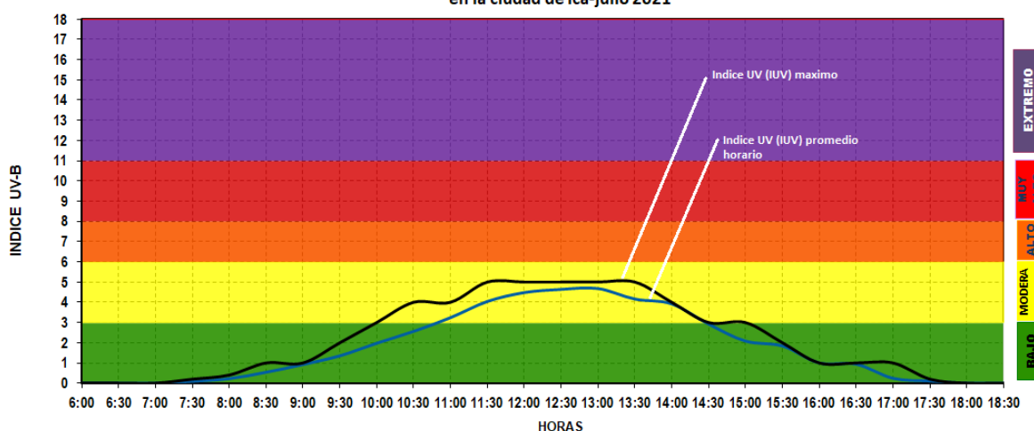
Fig.1: Índice horario de Radiación Solar Ultravioleta (IUV) en la ciudad de Ica-julio 2021
