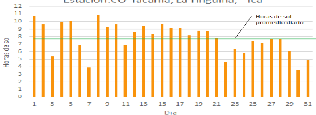
Fig.2: Horas de sol total diario mayo 2021 Estacion:CO Tacama, La Tinguña, Ica
