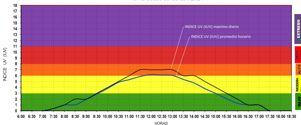
Fig.1: Índice promedio horario de Radiación Solar Ultravioleta (IUV) en la ciudad de Ica-abril 2021
