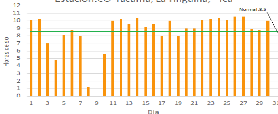
Fig.2: Horas de sol total diario abril 2021 Estacion:CO-Tacama, La Tinguiña, -Ica
