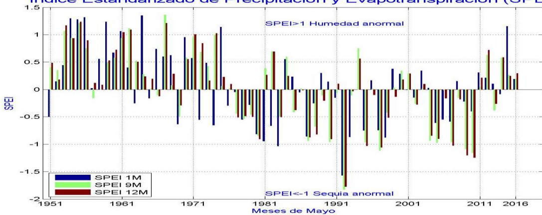
Serie temporal del SPEI sobre la región del recuadro (DZ4)
