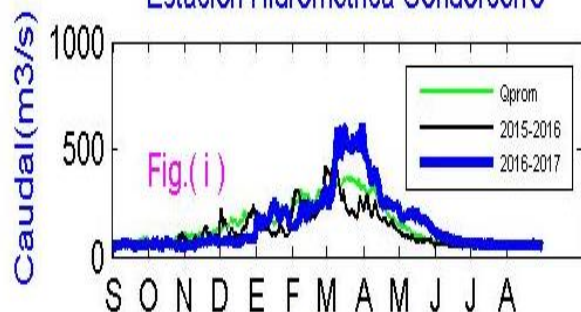
Hidrograma Río Santa Estación Hidrométrica Condorcero
