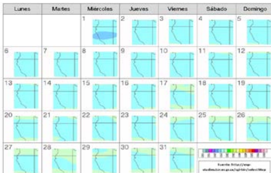
Mapa diario del ozono total atmosférico para el mes de agosto 2018
