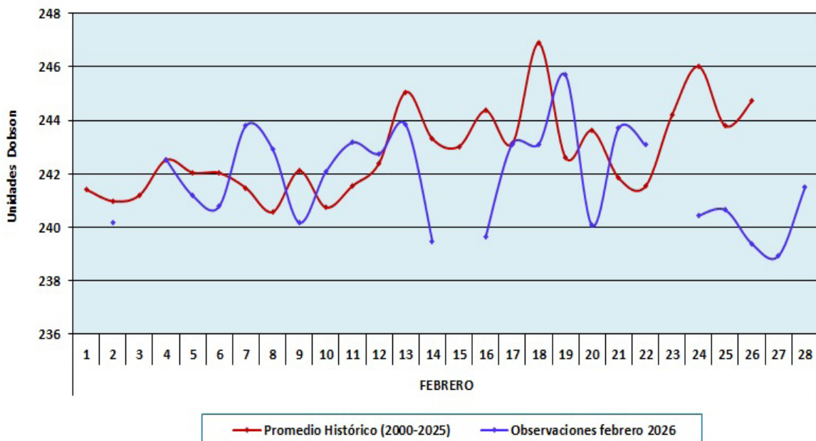
FIGURA N° 3 Comportamiento temporal de la concentración de ozono atmosférico en el OVA Marcapomacocha. Febrero 2026.
