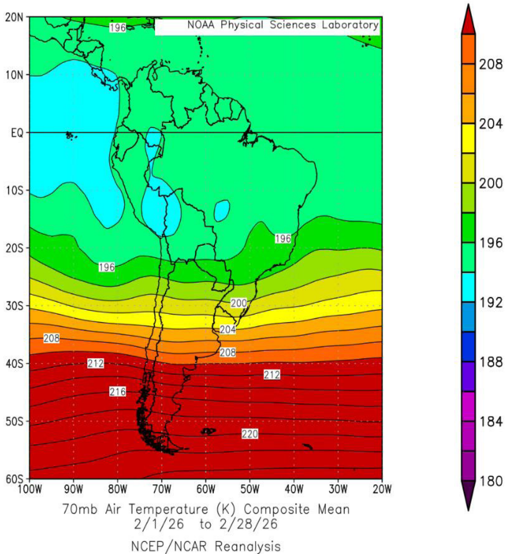
Comportamiento del régimen térmico en la baja estratósfera para el mes de febrero 2026
