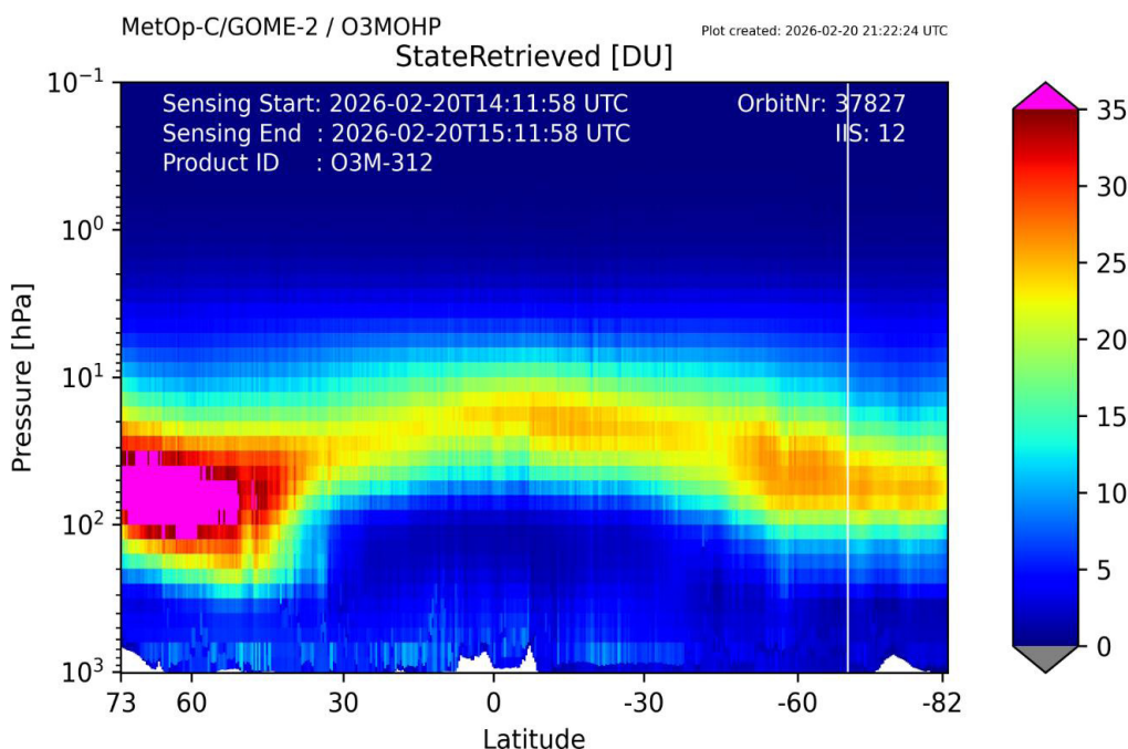
FIGURA N° 5 Perfil Vertical de Ozono según GOME-2 Fuente: Metop-C/GOME-2
