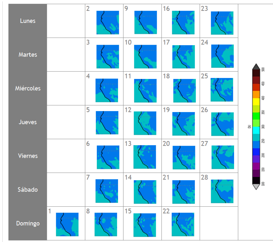
FIGURA N° 7 Mapa diario del ozono total atmosférico para el mes de febrero 2026 Fuente: Satélite AURA
