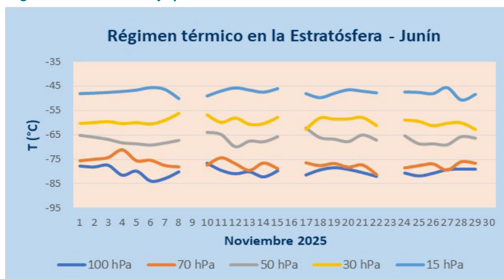
FIGURA N° 10 Régimen térmico en la baja y media estratósfera de Junín
