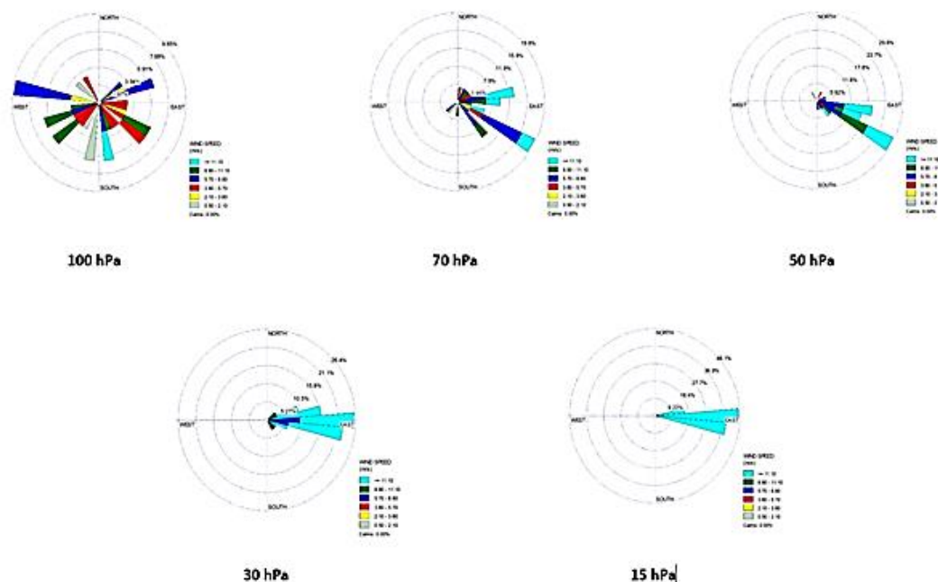
Comportamiento del viento en la baja y media estratósfera para el mes de marzo 2025
