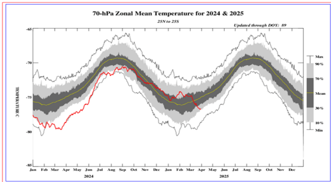
Comportamiento de la temperatura en la baja estratósfera para el mes de marzo 2025 Fuente: National Weather Service, Climate Prediction Center (Web Site)
