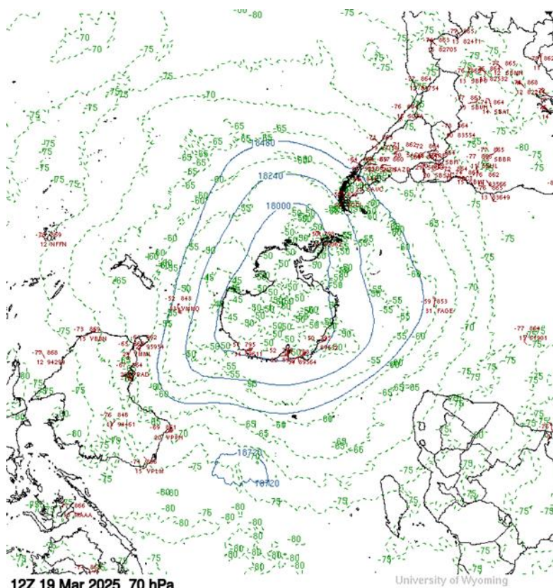
Comportamiento de la temperatura en 70 hPa para el hemisferio sur (19 marzo 2025)
