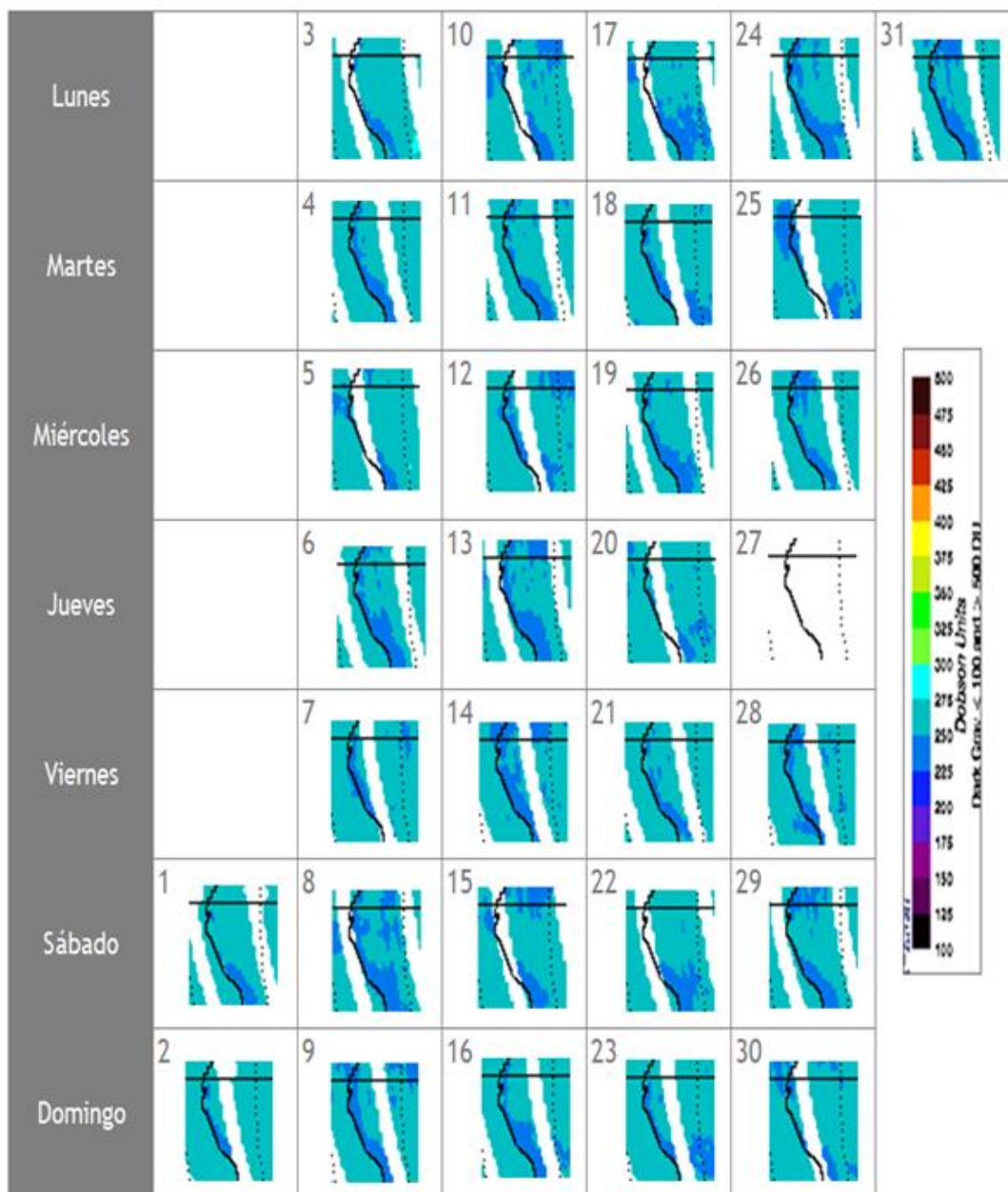
Mapa diario del ozono total atmosférico para el mes de marzo 2025
