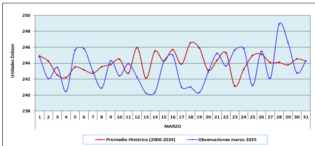
Comportamiento temporal de la concentración de ozono atmosférico en el OVA Marcapomacocha. Marzo 2025.
