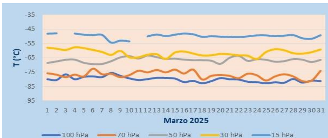
Régimen térmico en la baja y media estratósfera de Junín
