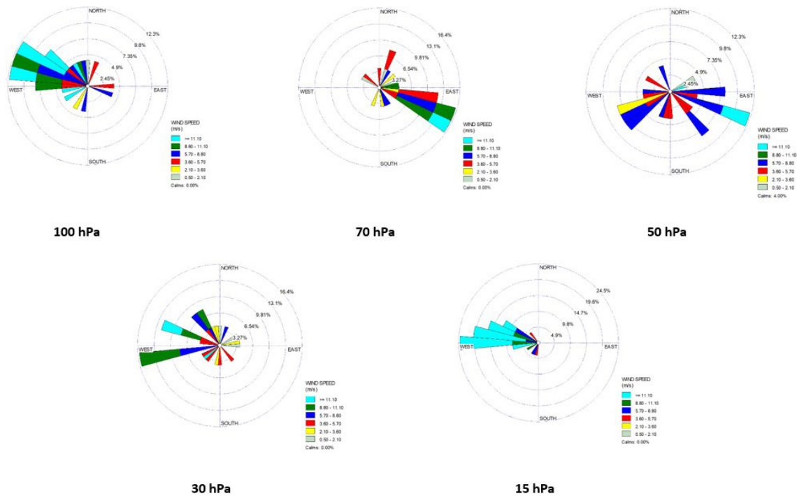
Comportamiento del viento en la baja y media estratósfera para el mes de agosto 2024
