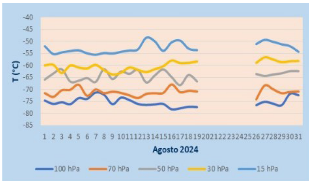
FIGURA N° 11 Régimen térmico en la baja y media estratósfera de Junín
