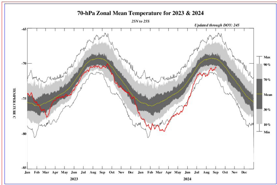
FIGURA N° 10 Comportamiento de la temperatura en la baja estratósfera para el mes de agosto 2024
