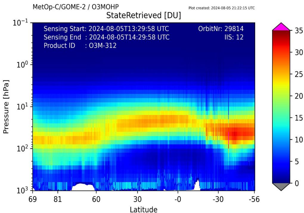
FIGURA N° 6 Perfil Vertical de Ozono según GOME-2
