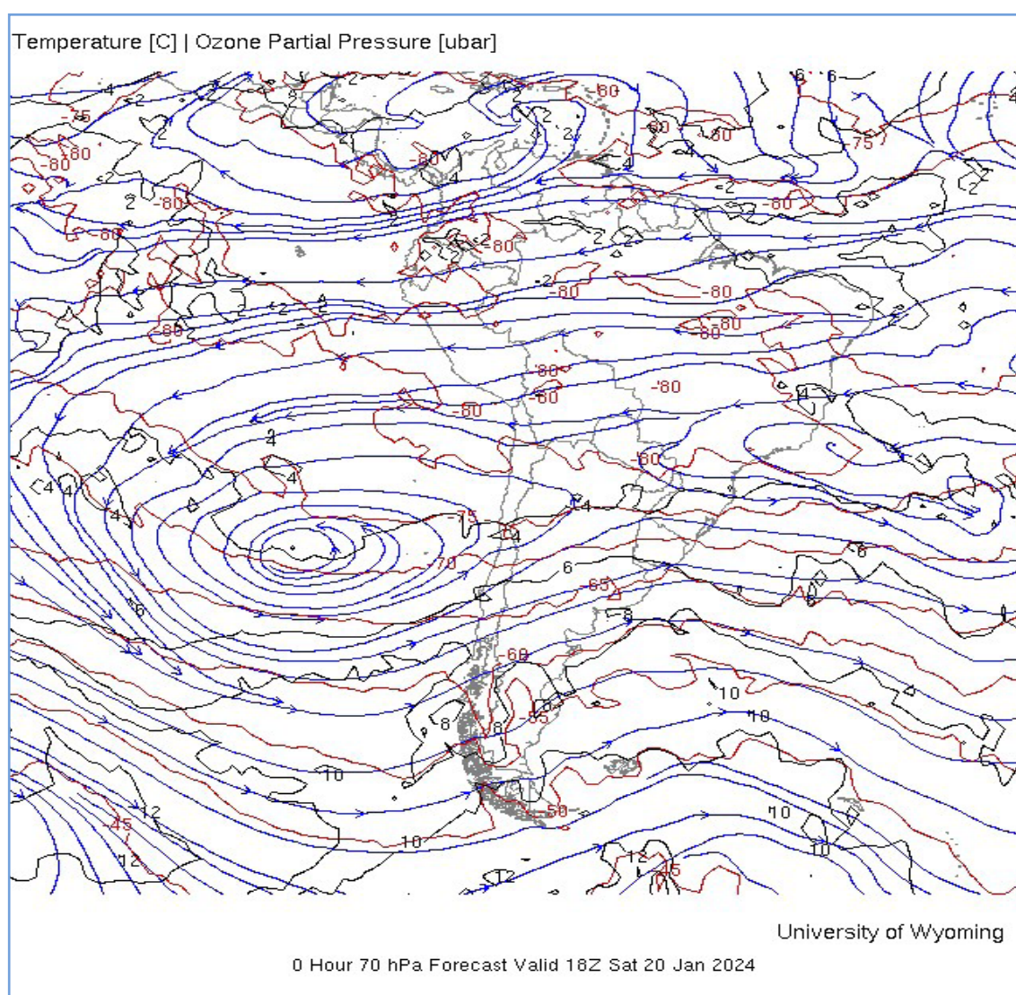
FIGURA N° 2 Flujos de masas de aires zonales
