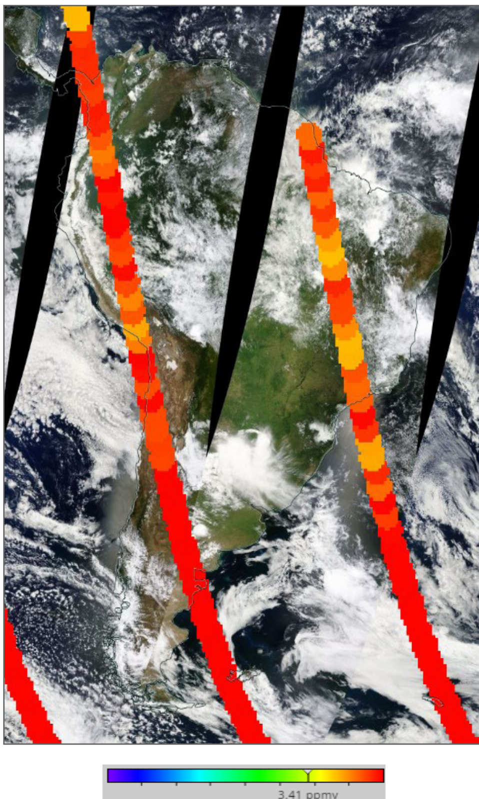
FIGURA N° 7 Vapor de Agua a 46 hPa
