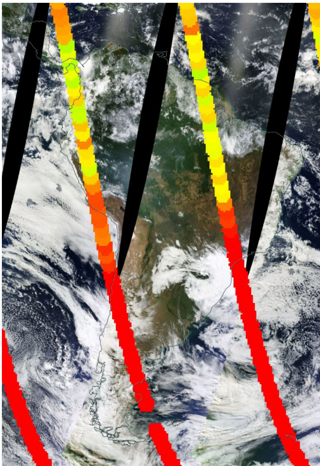
FIGURA N° 8 Vapor de Agua a 46 hPa
