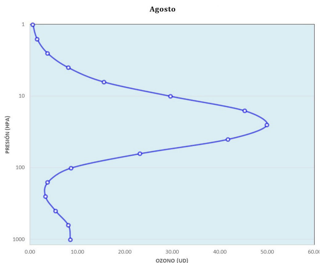
FIGURA N° 5 Perfil Vertical de Ozono OVA Marcapomacocha
