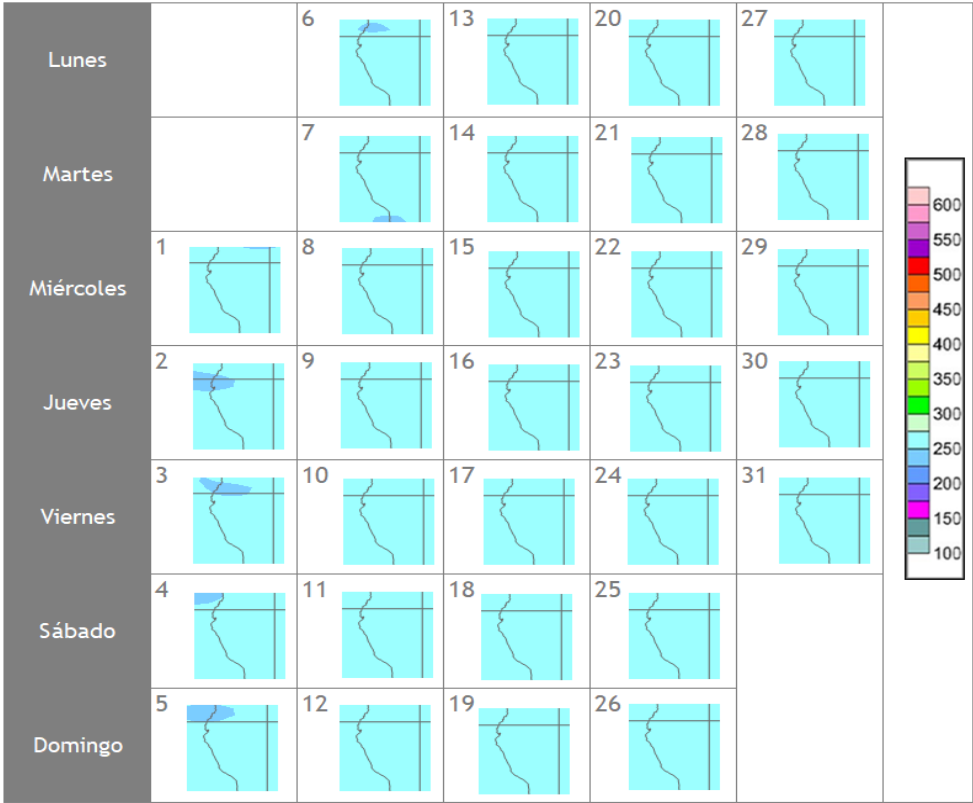
FIGURA N° 9 Mapa diario del ozono total atmosférico para el mes de marzo 2023
