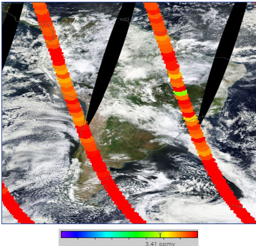
FIGURA N° 8 Vapor de Agua a 46 hPa
