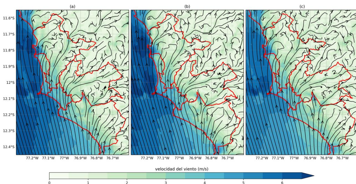
Figura N° 04. Decadriaria de líneas de corriente de la velocidad del viento (m/s) a 10m en el AMLC.
