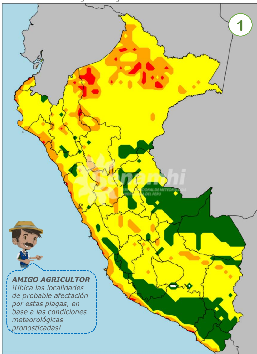
Mosca minadora
