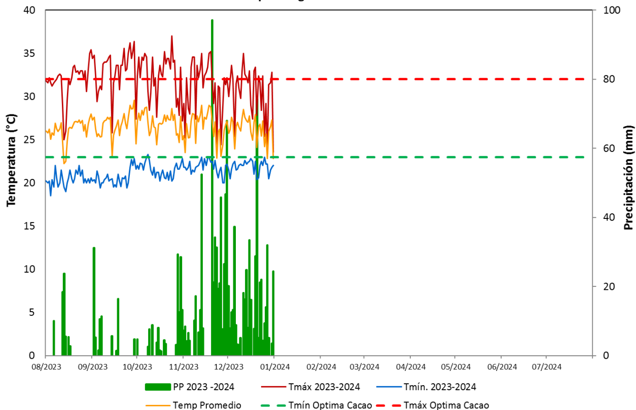
Gráfico 1: Régimen de precipitación y temperaturas extremas en Aucayacu (Huánuco)
