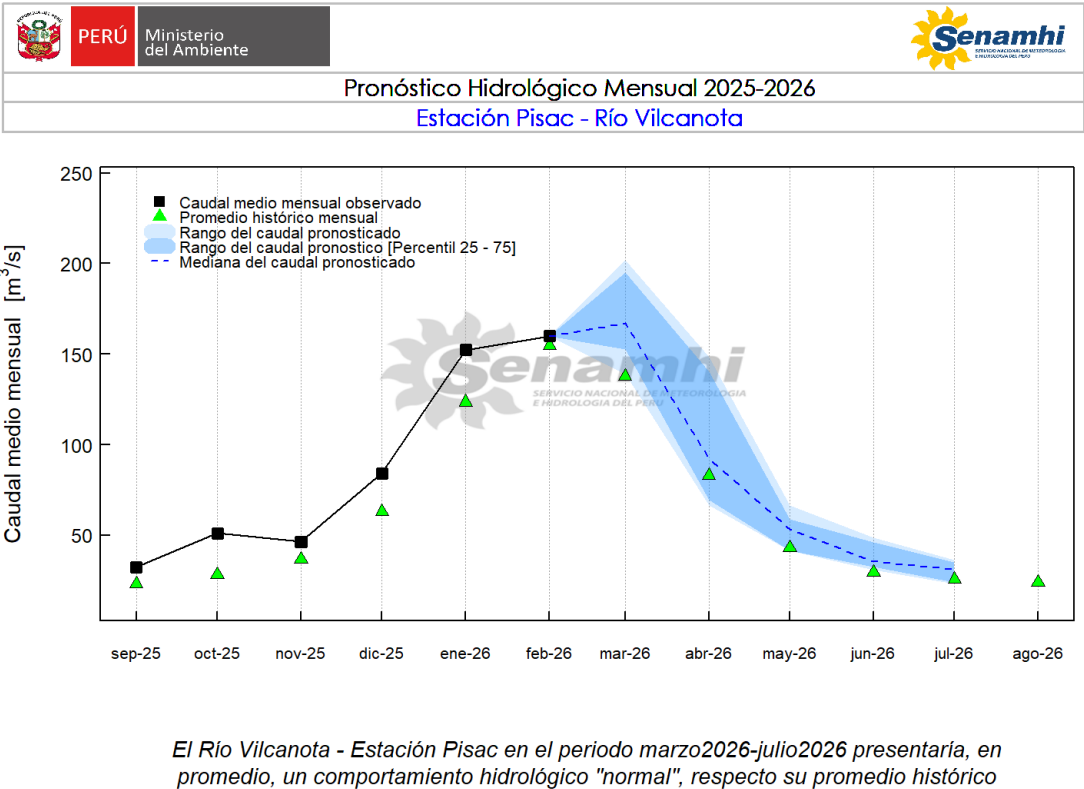
Figura 20. Pronóstico Hidrológico Estacional para la cuenca del río Vilcanota – Estación Pisac
