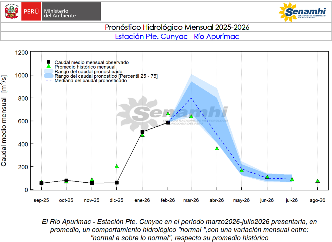
Figura 21. Pronóstico Hidrológico Estacional para la cuenca del río Apurímac – Estación Cunyac
