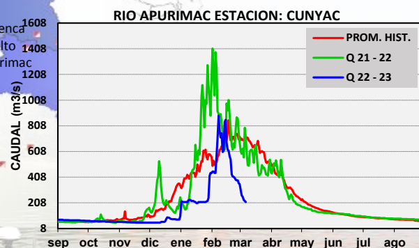
Figura 10 Caudales y niveles diarios de los ríos de la RHA zona centro y sur.
