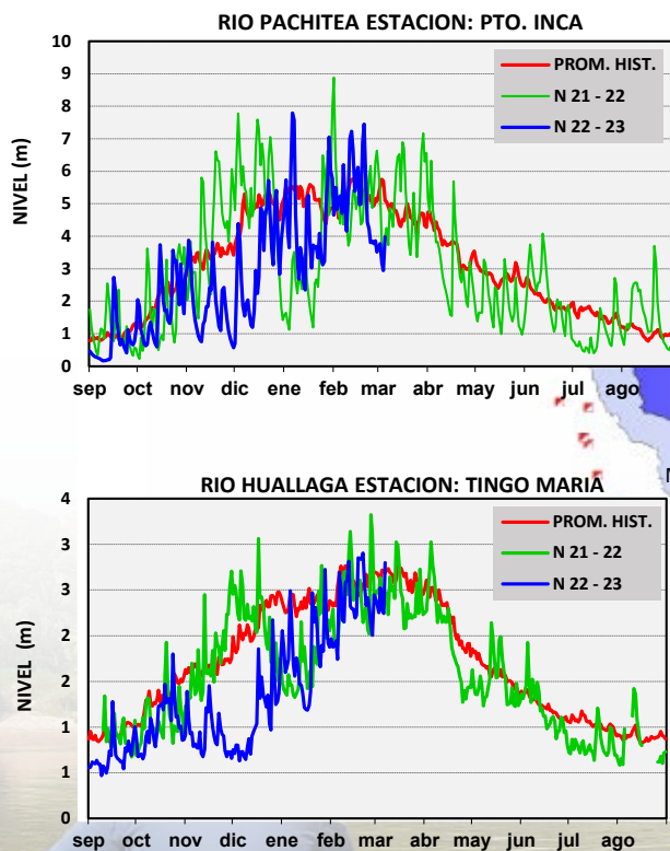
Figura 10 Caudales y niveles diarios de los ríos de la RHA zona centro y sur.
