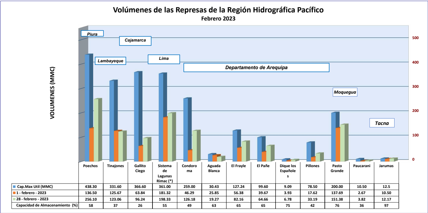
Figura 6 Volúmenes de almacenamiento en la región hidrográfica Pacífico
