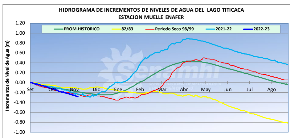
Figura 7 Variación de los niveles del agua del Lago Títicaca
