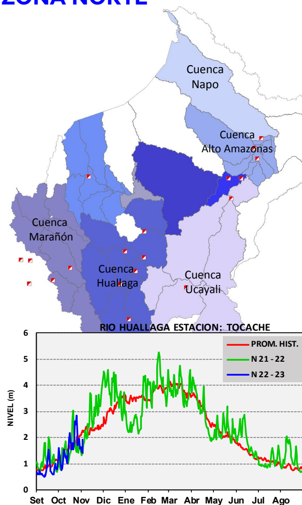
Figura 8 Niveles diarios de los ríos de la RHA zona norte
