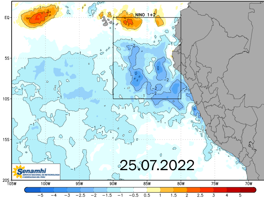
SENAMHI/DMA/SPM OSTIA - ANOMALIA DE LA TEMPERATURA SUPERFICIAL DEL MAR (°C) 25 de Julio de 2022
