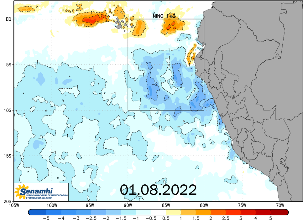
SENAMHI/DMA/SPM OSTIA - ANOMALIA DE LA TEMPERATURA SUPERFICIAL DEL MAR (°C) 01 de Agosto de 2022
