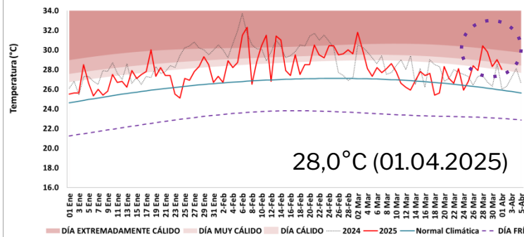
TEMPERATURA MÁXIMA [°C] ESTACIÓN: VON HUMBOLDT - LIMA - LA MOLINA
