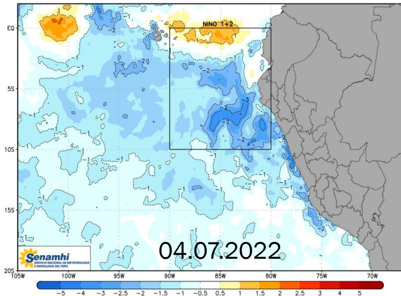
SENAMHI/DMA/SPM OSTIA – ANOMALIA DE LA TEMPERATURA SUPERFICIAL DEL MAR (°C) 04 de Julio de 2022
