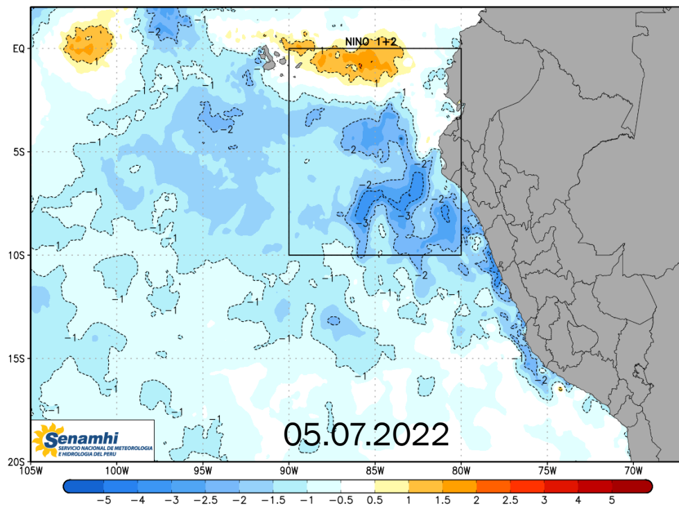
SENAMHI/DMA/SPM OSTIA – ANOMALIA DE LA TEMPERATURA SUPERFICIAL DEL MAR (°C) 05 de Julio de 2022
