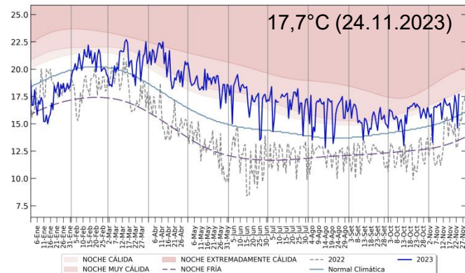
TEMPERATURA MÍNIMA [°C] ESTACIÓN: VON HUMBOLDT - LIMA
