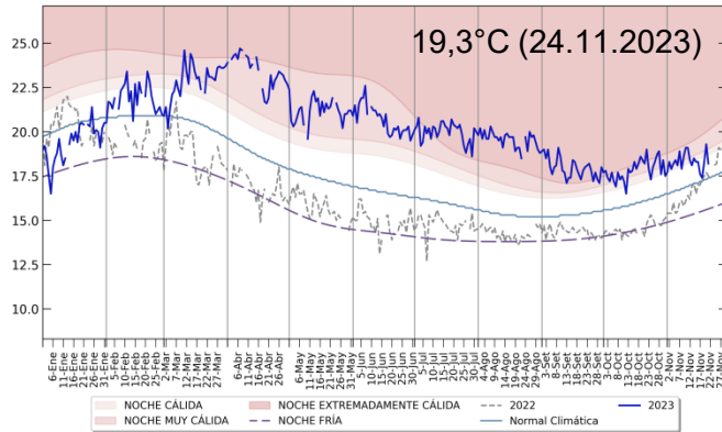
TEMPERATURA MÍNIMA [°C] ESTACIÓN: AEROPUERTO INTERNACIONAL - CALLAO
