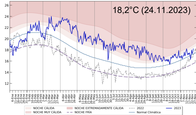
TEMPERATURA MÍNIMA [°C] ESTACIÓN: CAMPO DE MARTE - LIMA
