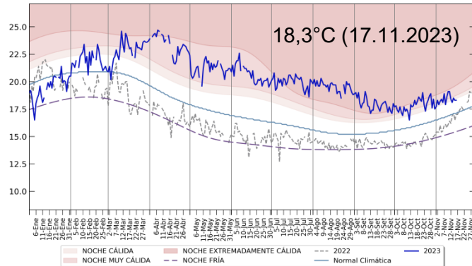
TEMPERATURA MÍNIMA [°C] ESTACIÓN: AEROPUERTO INTERNACIONAL - CALLAO
