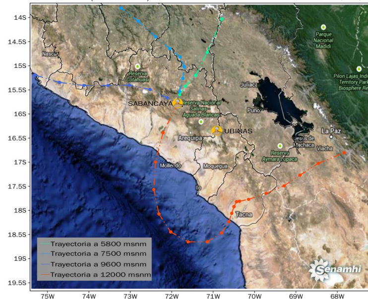
SUBDIRECCION DE MODELAMIENTO NUMERICO DE LA ATMOSFERA TRAYECTORIAS DE UNA PARCELA DE AIRE MODELO WRF (SABANCAYA) Valido: 7am - 07/FEB/2022
