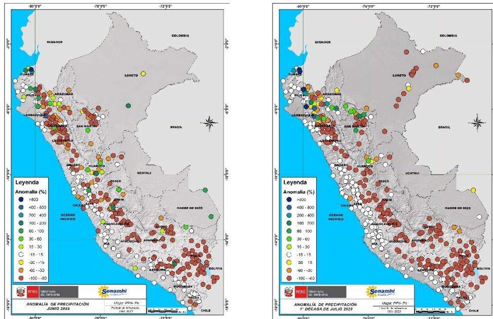
Figura 13. Anomalia porcentual (%) de la precipitación en junio (izquierda) y en los primeros 10 días de julio (derecha). Climatología 1991-2020. Fuente y Procesamiento: Senamhi.
