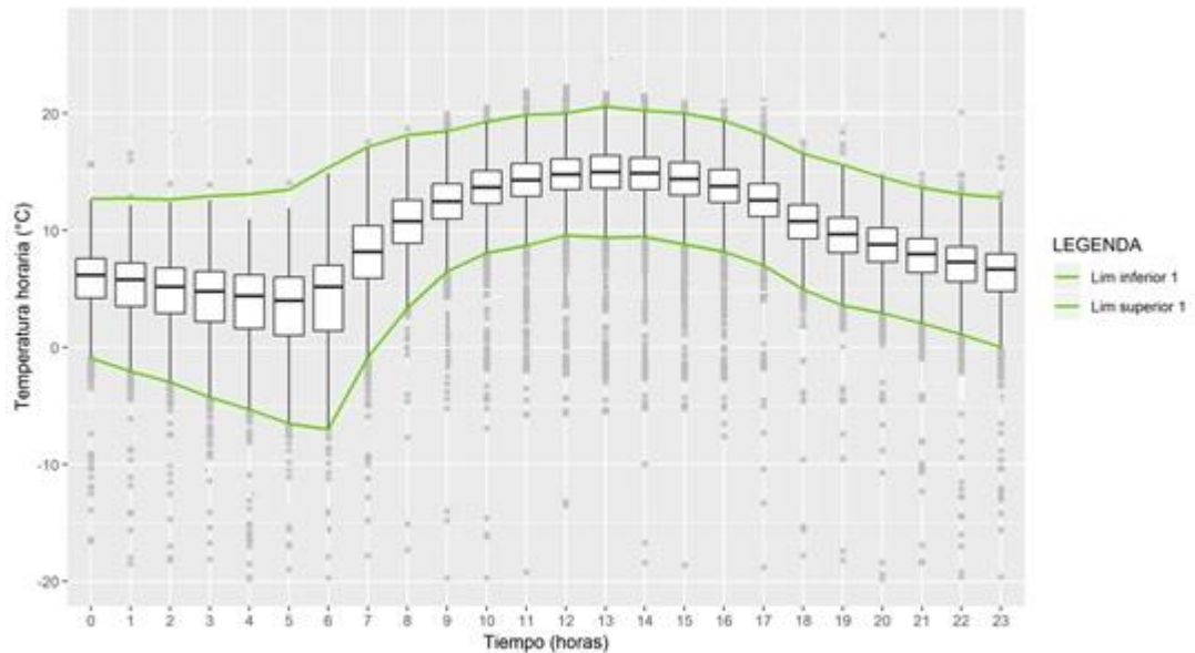
Figura: Límite máximo y mínimo horarios de la Temperatura del aire de la Estación Puente Carretera – Puno
