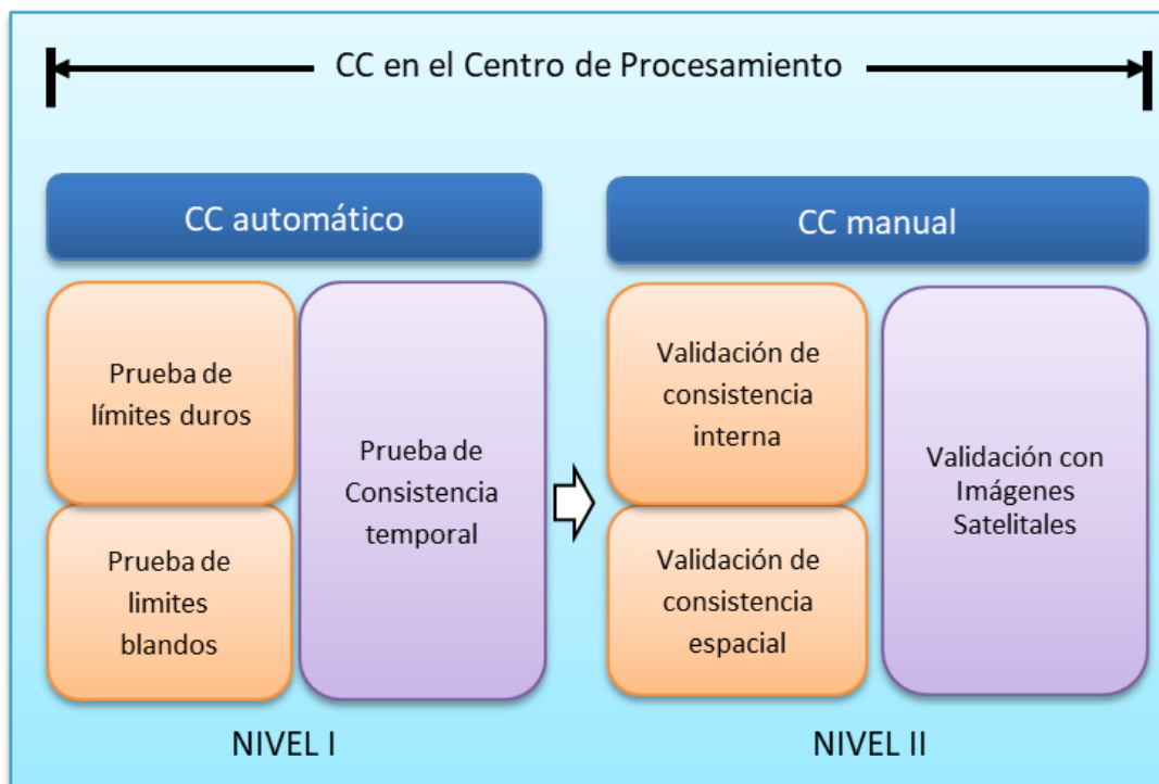
Figura N° 1: Flujograma de los procesos de Control de Calidad (CC) de los datos meteorológicos e hidrológicos de estaciones automáticas en el centro de procesamiento de datos del Senamhi.
