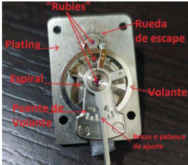
Volante del sistema de relojería con brazo o palanca de ajuste
