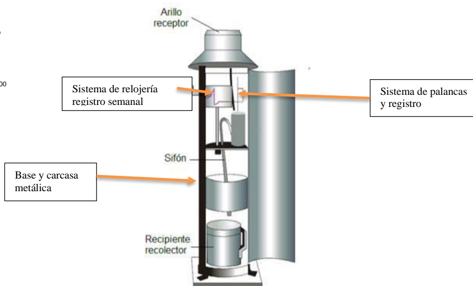
Figura N° 01. PLUVIOGRAFO 1507
