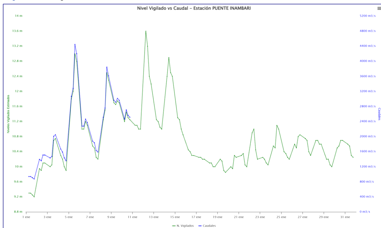
Figura 19. Hidrograma estación Río Inambari mes de enero del 2025
