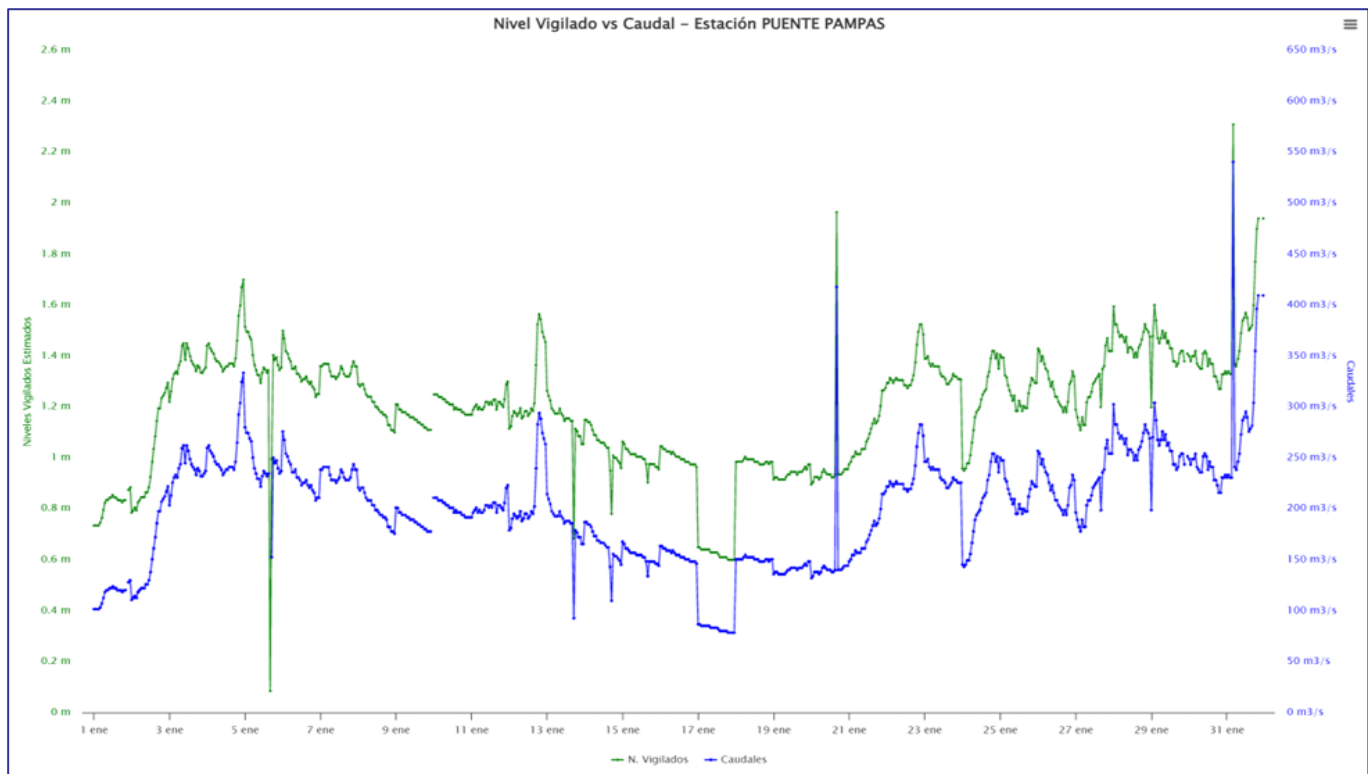
Figura 17. Hidrograma estación Puente Pampas mes de enero del 2025
