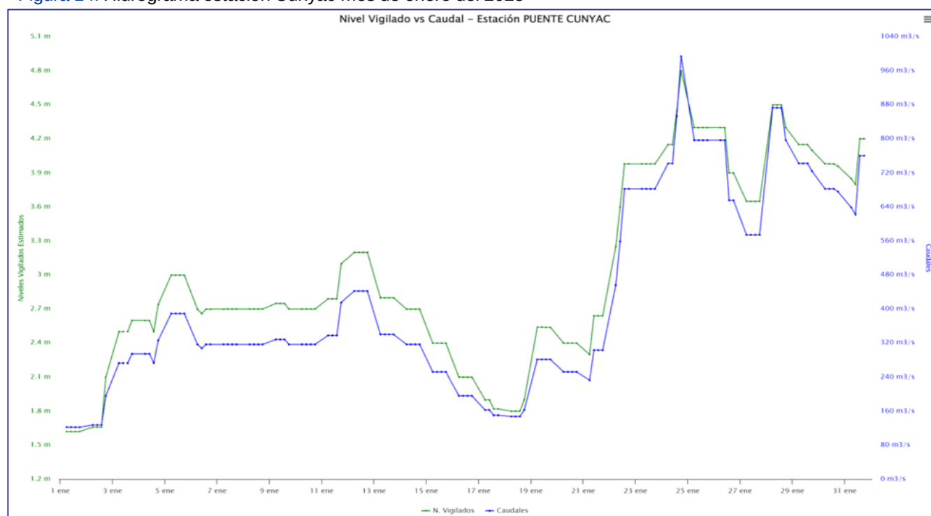
Figura 14. Hidrograma estación Cunyac mes de enero del 2025
