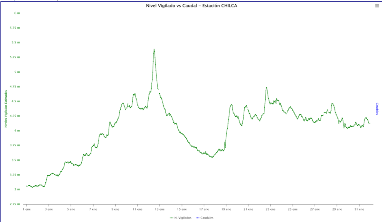
Figura 9. Hidrograma estación Chilca mes de enero del 2025
