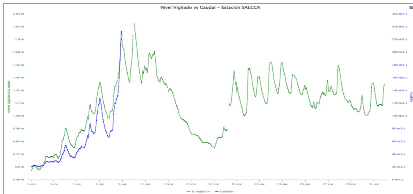
Figura 7. Hidrograma estación Salcca mes de enero del 2025
