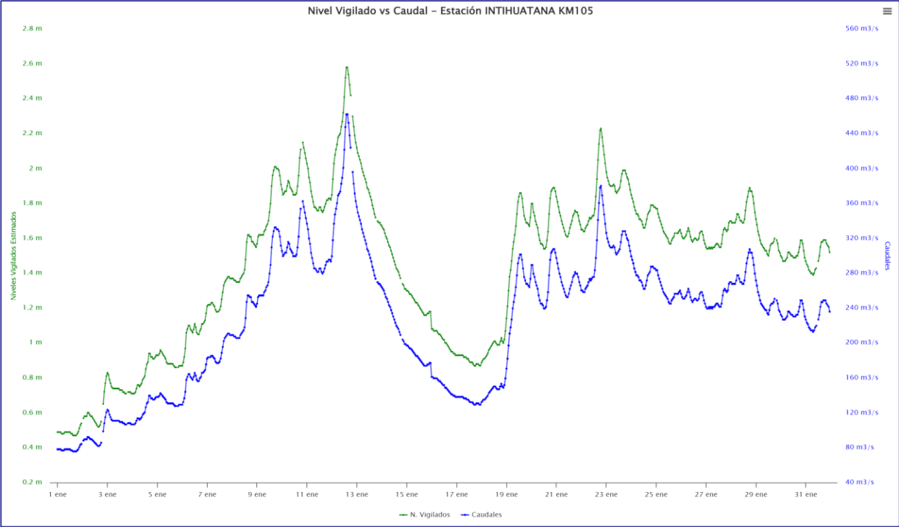
Figura 10. Hidrograma estación Intihuatana km 105 mes de enero del 2025
