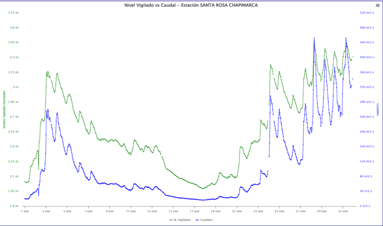
Figura 15. Hidrograma estación Santa Rosa mes de enero del 2025
