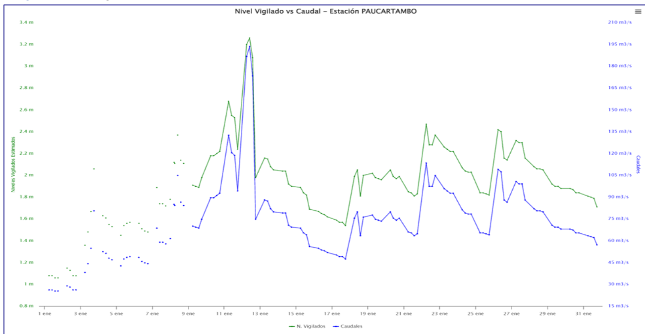
Figura 12. Hidrograma estación Paucartambo mes de enero del 2025
