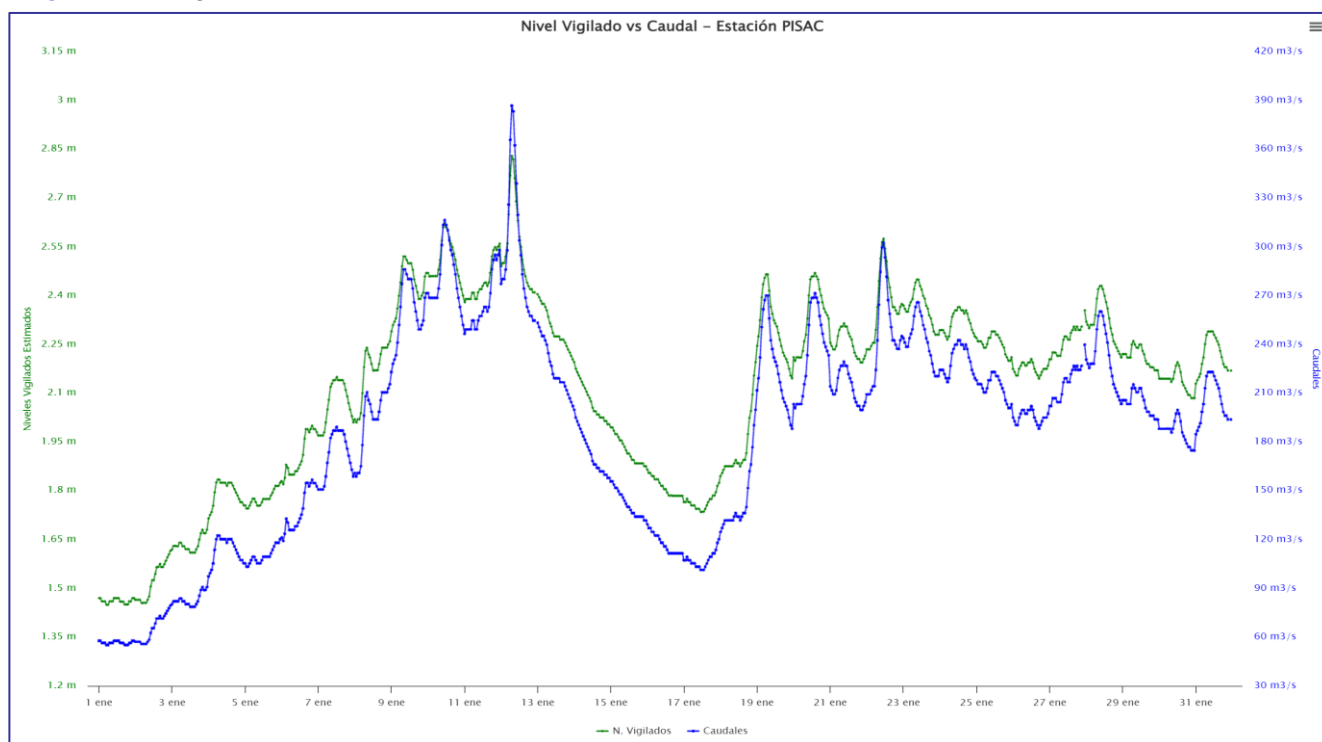
Cuadro 7: Caudales estación Pisac
