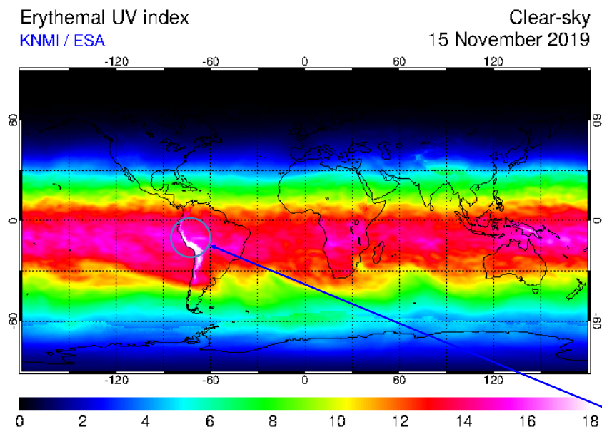
Figura N°2: Erythemal UV Index, Noviembre 2019
