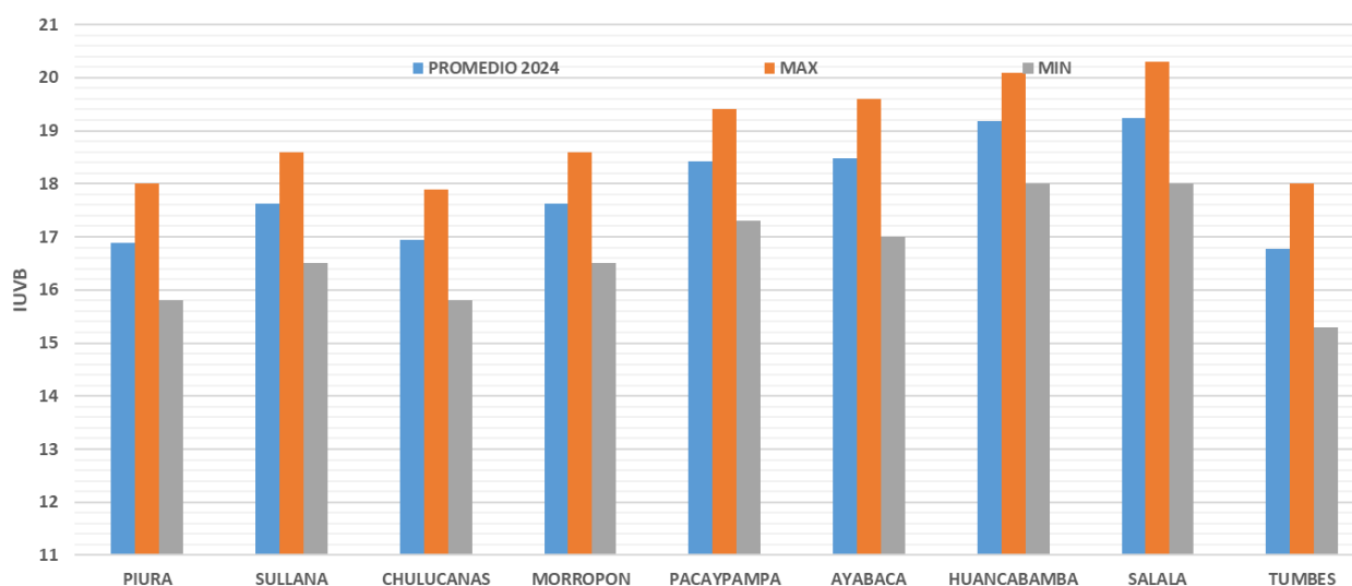
Fig 3. Distribución promedio máximo, medio y mínimo mensual correspondiente al mes de febrero, 2024 según provincias de las regiones Piura y Tumbes
