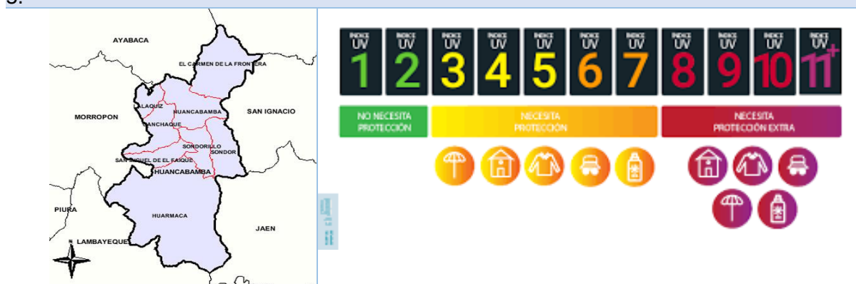
Fig. 5. Valor: promedio, máximo y mínimo de radiación ultravioleta ciudad de Huancabamba, mes de noviembre, 2022.
