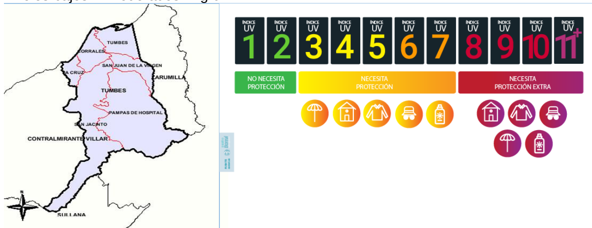
Fig.6. Valor: promedio, máximo y mínimo de radiación ultravioleta ciudad de la Cruz, mes de noviembre, 2022.
