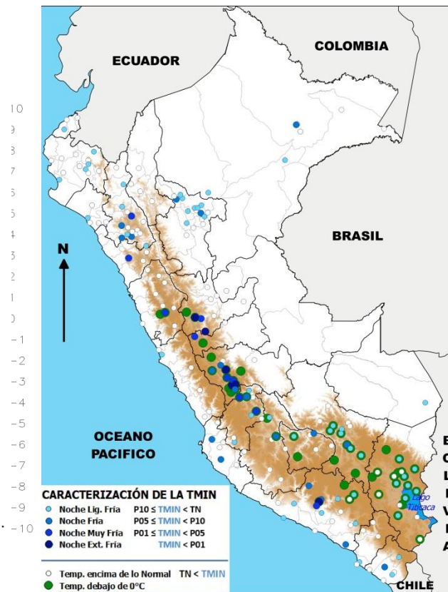
VARIACION DIARIA DE TEMPERATURA MINIMA 22JUL2017-21JUL2017
