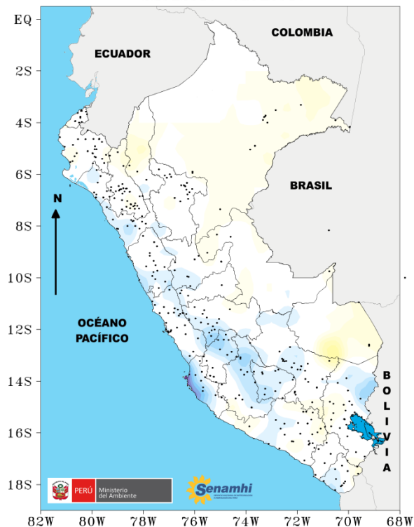
VARIACION DIARIA DE TEMPERATURA MINIMA 22JUL2017-21JUL2017
